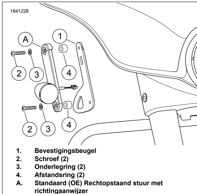
Afbeelding 2. Bevestigingsbeugel verwijderen/installeren (rechterkant afgebeeld)
