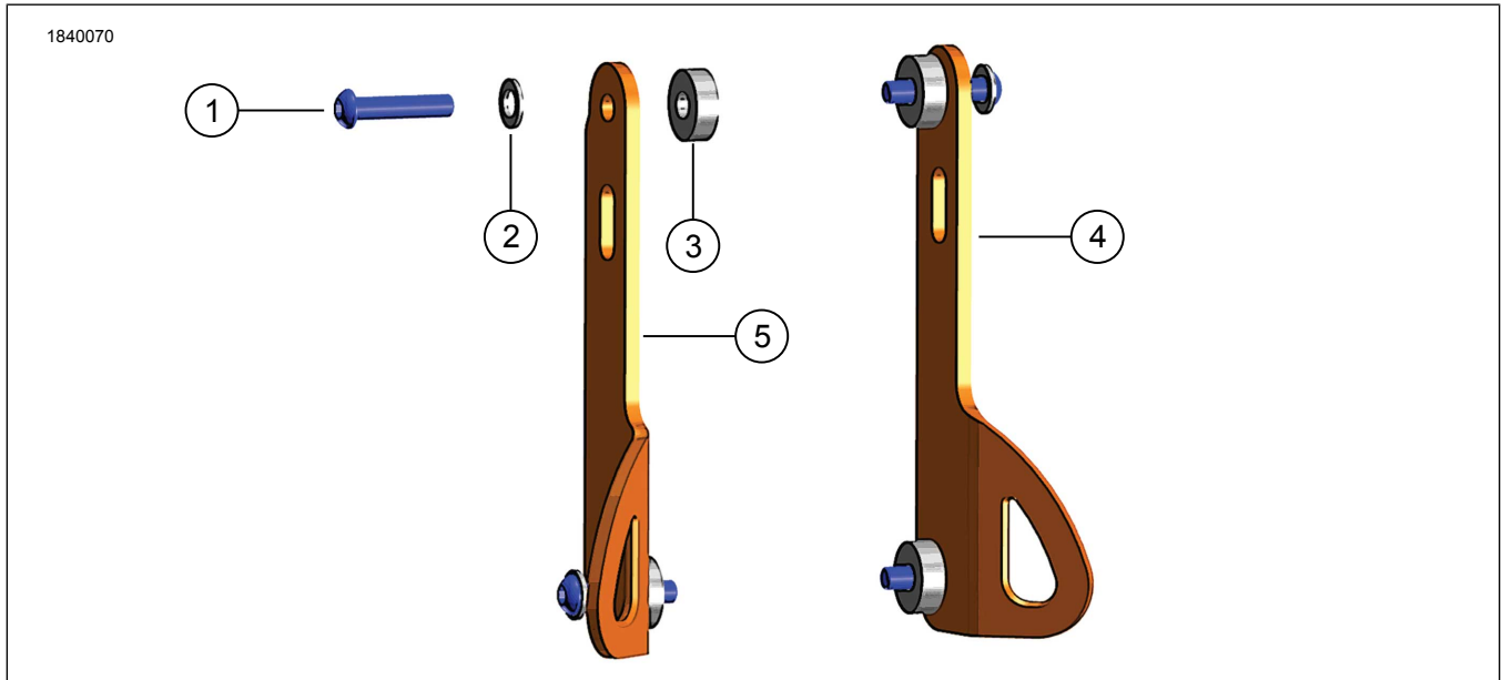
Figure 1. Contenu du kit : Supports d'arrimage
