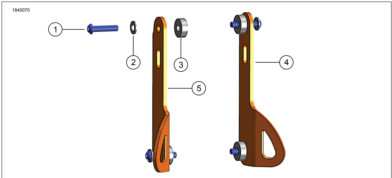
Figura 1. Conteúdo do kit: Suportes de Amarração
