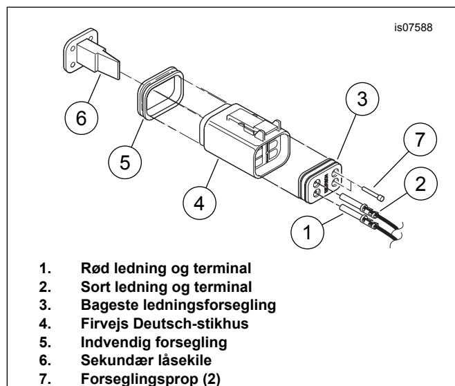
Figur 4. Sæt terminaler i Deutsch-stikhuset
