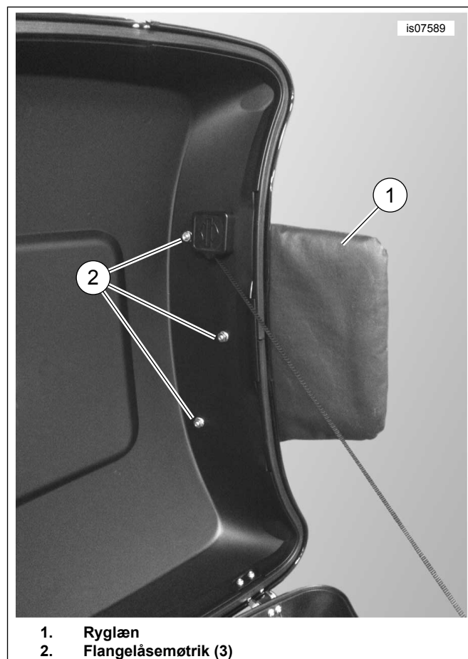
Figur 5. Monteret beslag på hakket Tour-Pak låg
