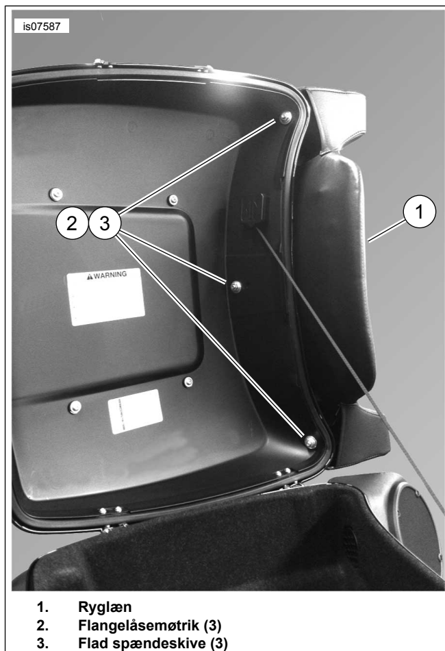
Figur 3. Monteret ryglæn på King Tour-Pak-låg
