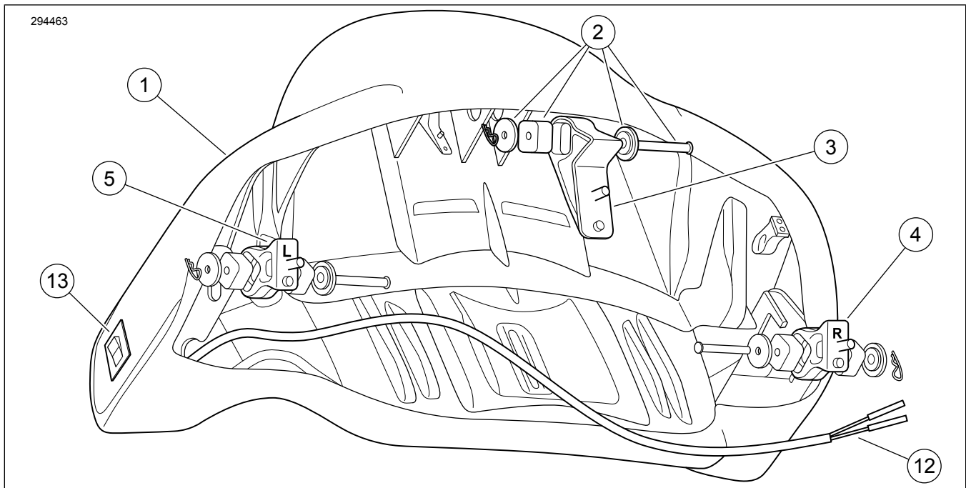
Figur 1. Sættets indhold: King Tour-Pak ryglæn sæt 52300312, 52300314, 52300316, 52300317, 52300334, 52300574, 52300744
