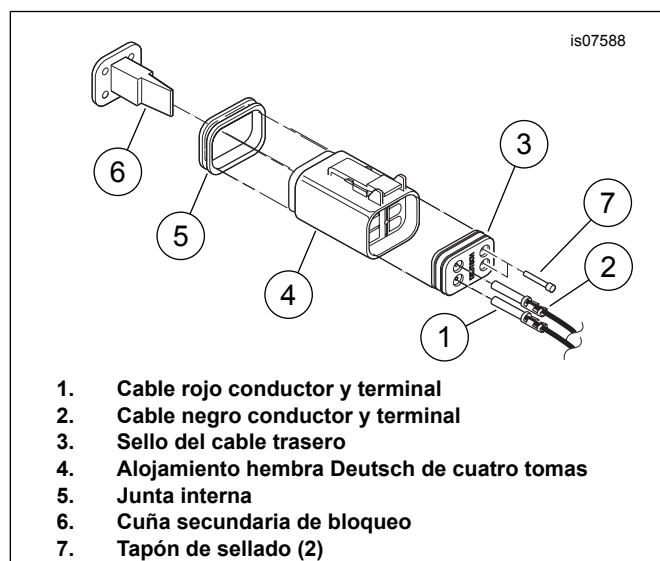
Figura 4. Inserte las terminales en el alojamiento del conector hembra Deutsch
