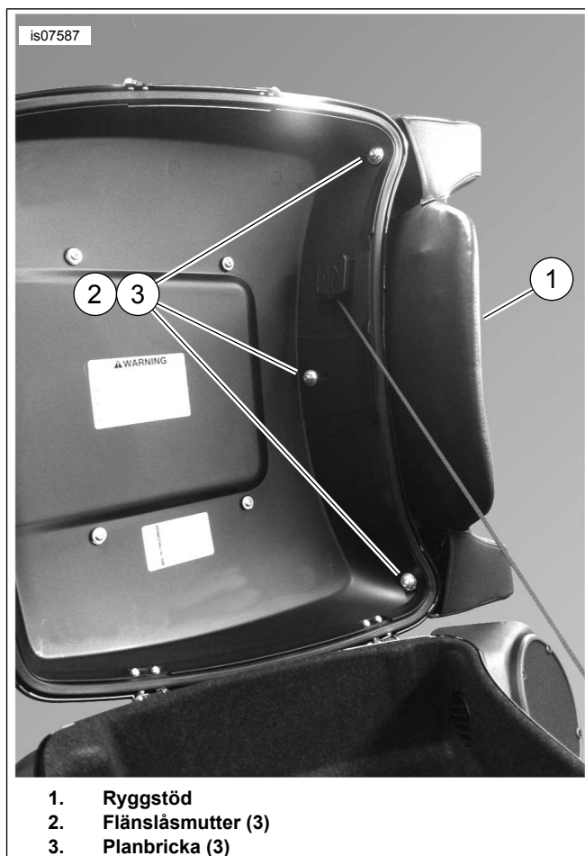
Figur 3. Monterat ryggstöd på King Tour-Pak-locket
