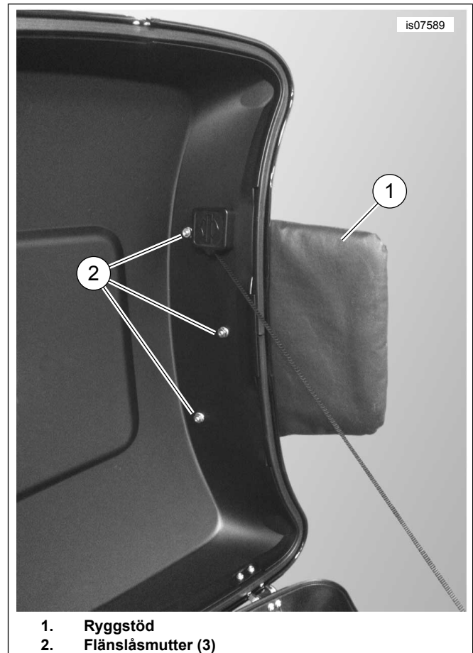
Figur 5. Monterat ryggstöd på det avkapade Tour-Pak-locket
