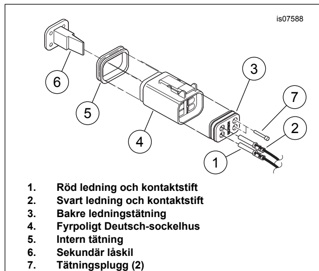
Figur 4. Sätt i kontaktstiften i Deutsch-uttagshuset
