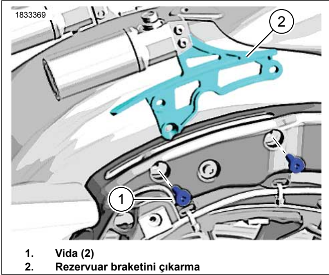
Şekil 2. Uzak Rezervuar Braketini Çıkarma
