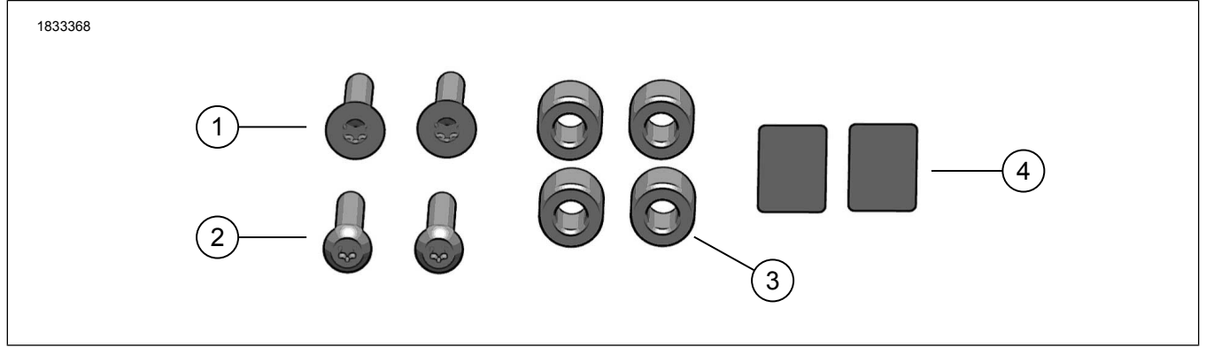
Şekil 1. Kit İçerikleri: Çıkarılabilir Dönüştürme Donanımı
