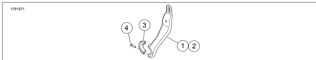
Figure 1. Contenu du kit : Kit de support de carénage
