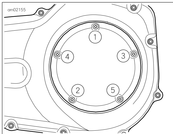
圖2。離合器蓋旋緊順序
