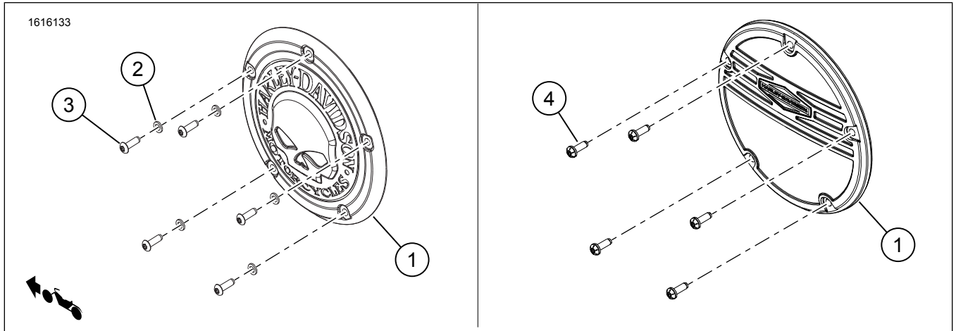
圖1。套件內容：Derby 蓋部件
