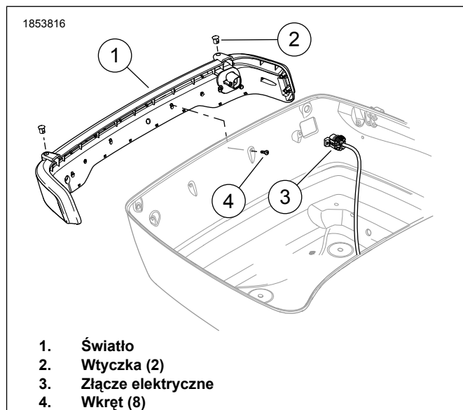
Rysunek 3. Lampa profilowana (typowa)
