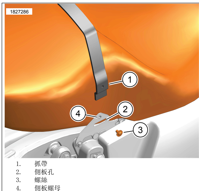
圖4。座椅抓帶安裝
