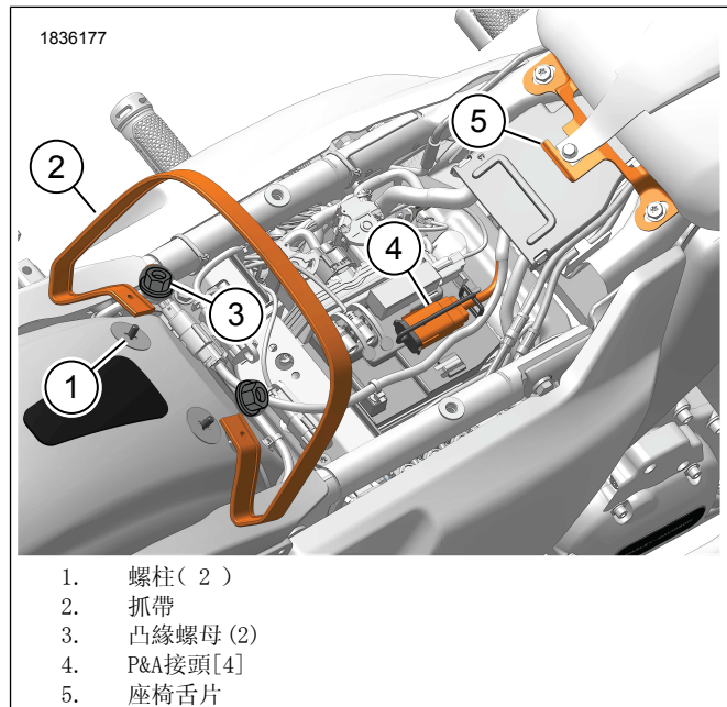
圖3。組件位置
