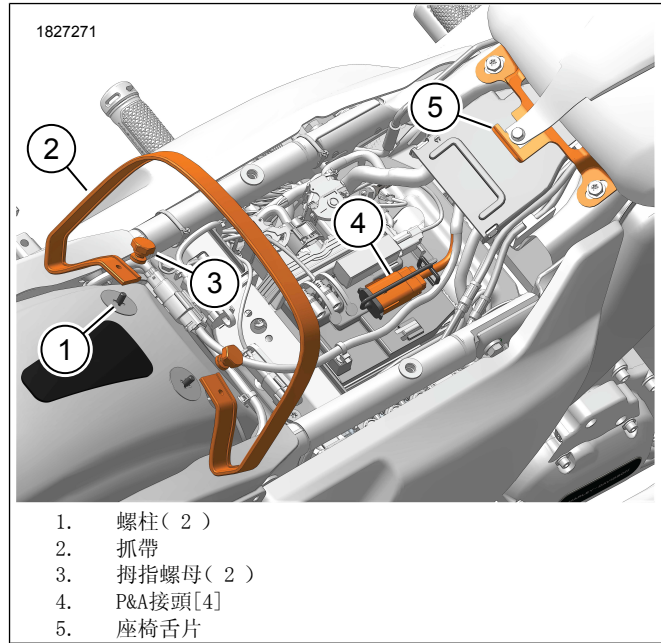
圖2。組件位置
