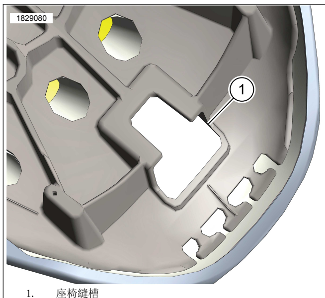
圖5。座椅安裝槽
