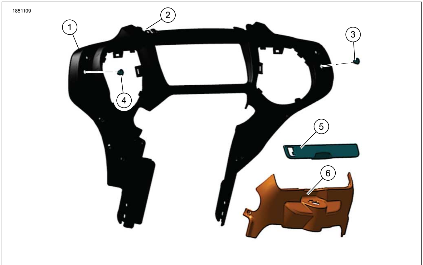
Figure 1. Contenu du kit : Carénage interne
