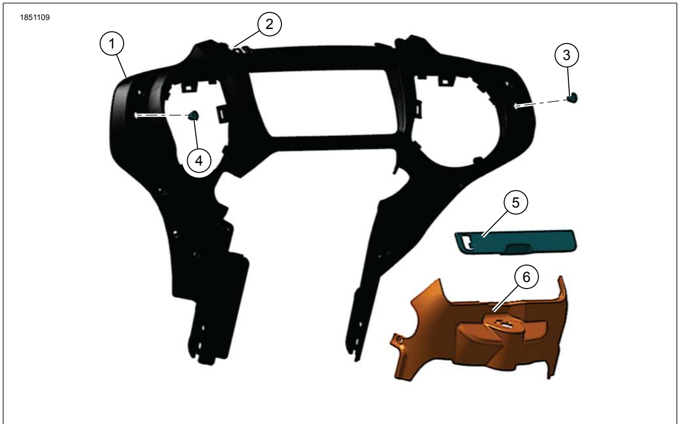
Figure 1. Contenu du kit : Carénage intérieur
