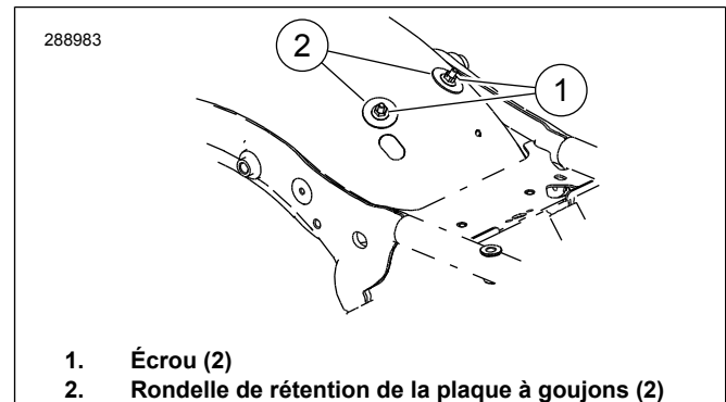
Figure 1. Enlevez les écrous
