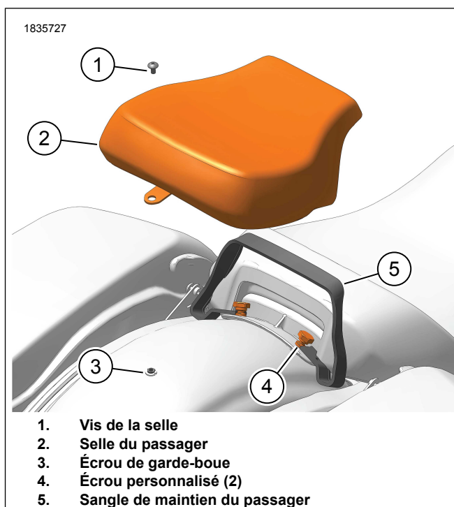
Figure 2. Installation de la selle du passager
