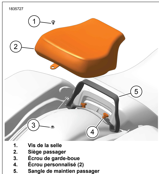
Figure 2. Installation du siège passager
