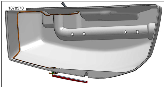
圖6。線束佈設
