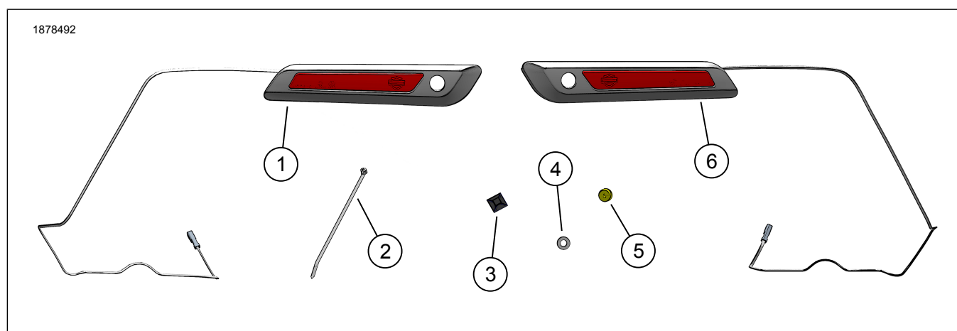
Figur 1. Sættets indhold: Sadeltaske sidemarkering lampesæt
