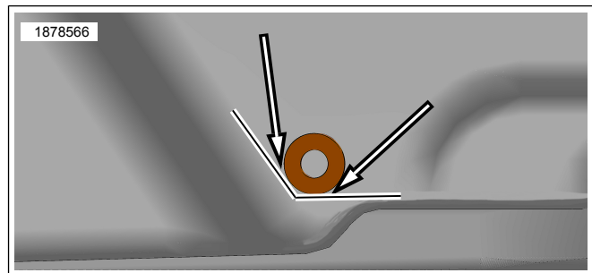
Figur 5. Sadeltaske Nedre hul Drill Placering
