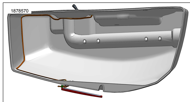
Figur 6. Ledningsnetføring
