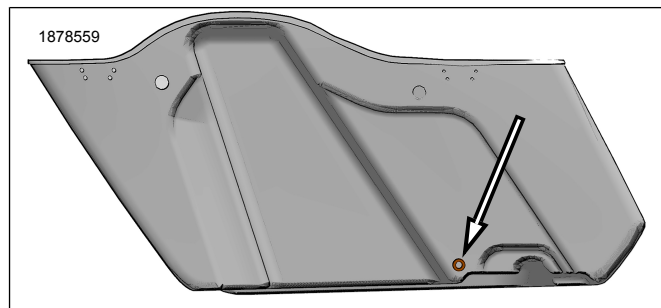
Figur 4. Sadeltaske Nedre hul Drill Placering
