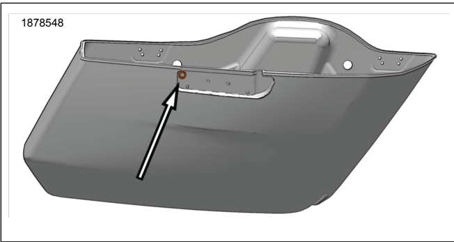
그림 2. 새들백 상단 구멍 드릴 위치
