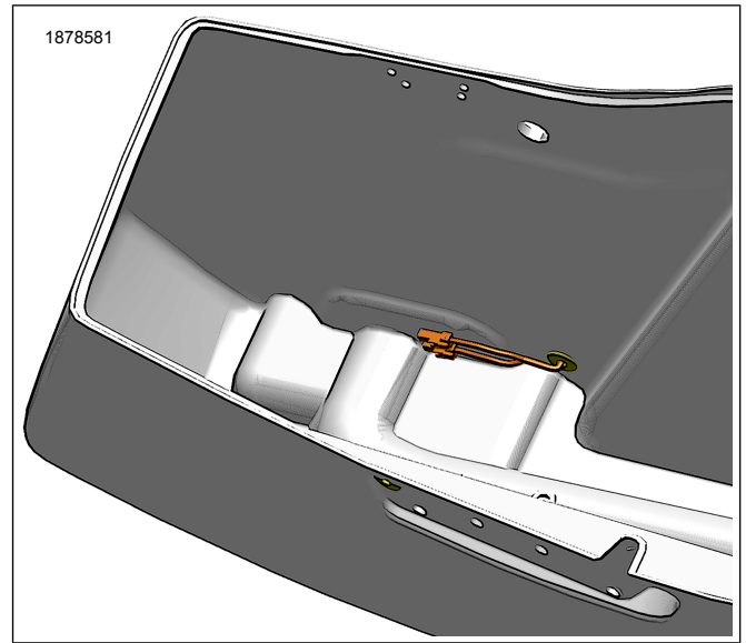
그림 7. 점퍼 하네스 배선(설치된 경우)
