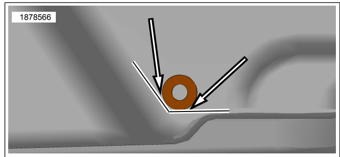
그림 5. 새들백 하부 구멍 드릴 위치
