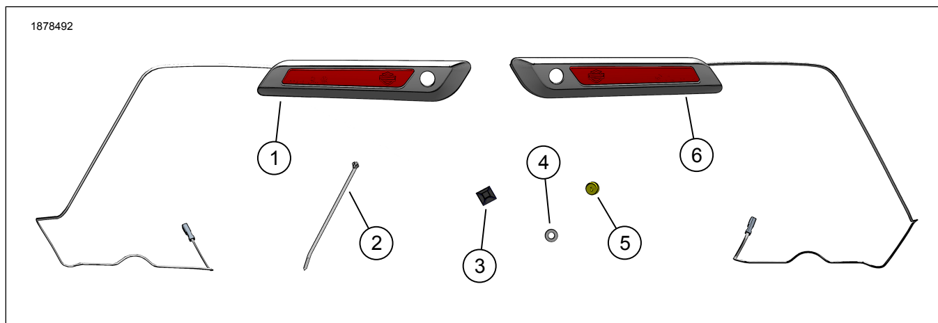
図1。キット内容: サドルバッグサイドマーカーランプキット
