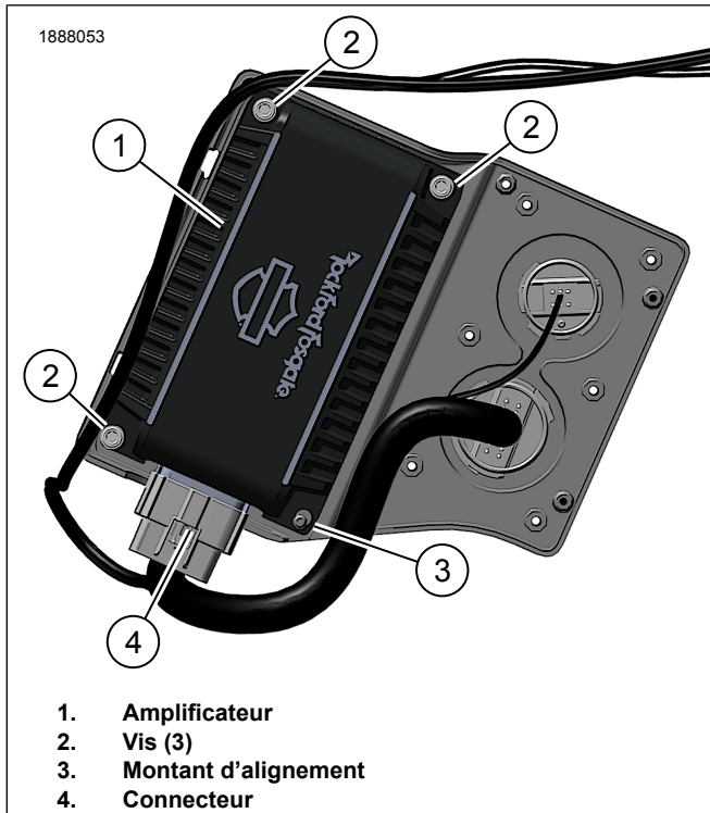
Figure 3. Amplificateur (secondaire)
