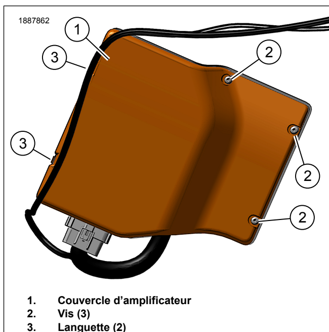
Figure 2. Couvercle de l'amplificateur (secondaire)
