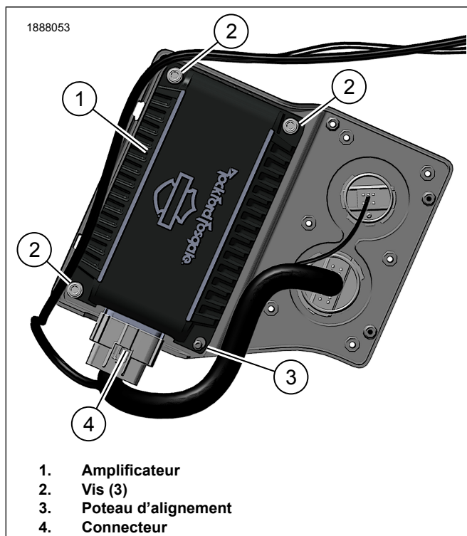
Figure 3. Amplificateur (secondaire)
