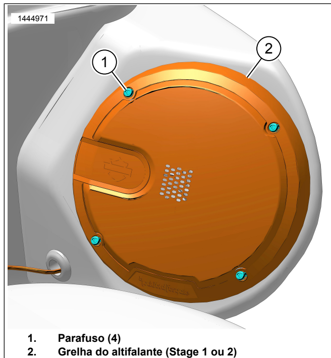
Figura 3. Grelha da Cápsula do Altifalante (Vista do Lado Esquerdo)
