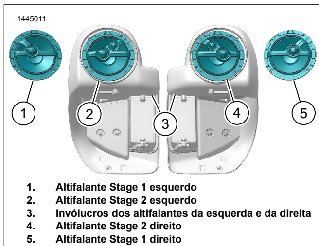
Figura 2. Orientação de Altifalantes com Arrefecimento a Ar
