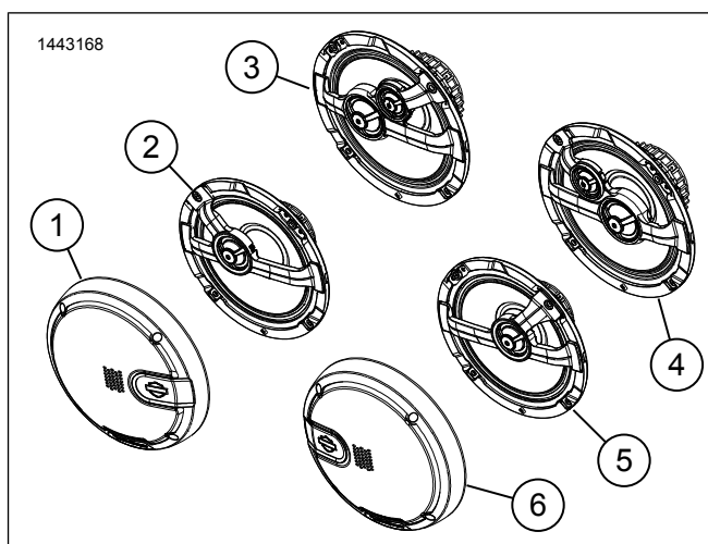
Afbeelding 4. Serviceonderdelen, Boom! Audio 165 mm (6,5 in) luidsprekerset achter
