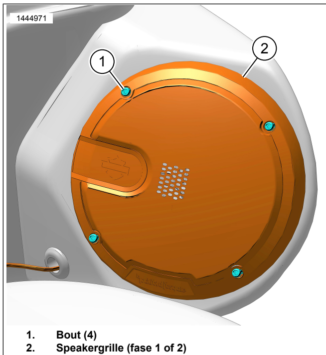
Afbeelding 3. Luidsprekerhuls (links getoond)
