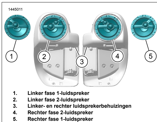
Afbeelding 2. Oriëntatie luchtgekoelde luidspreker
