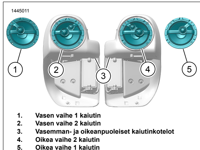
Kuva 2. Ilmajäähdytteisten kaiutinten suuntaus
