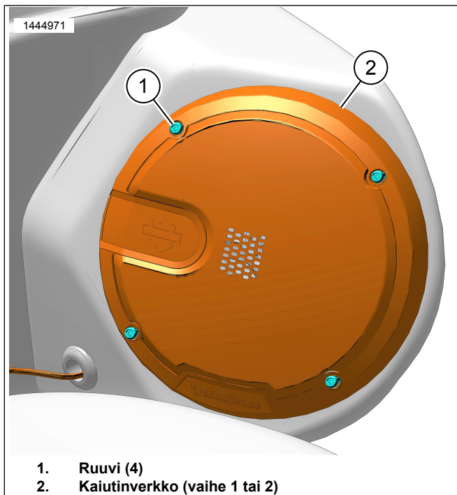
Kuva 3. Kaiutinkotelon suojaritilä (vasenpuoli kuvassa)
