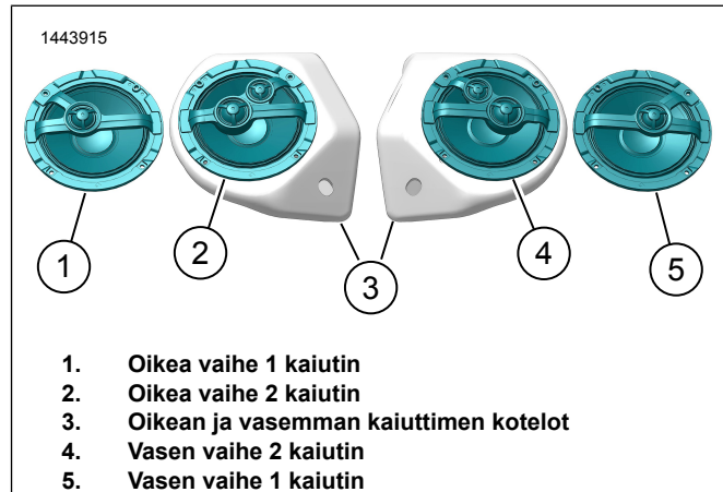
Kuva 1. Tour-Pak-kaiutinten suuntaus
