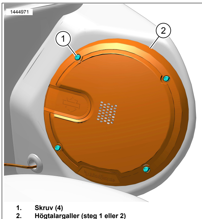
Figur 3. Högtalargaller (vänster sida visad)
