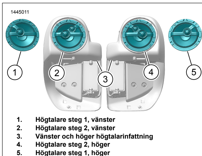
Figur 2. Orientering av högtalare på luftkylda modeller
