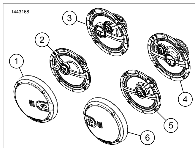
Figur 4. Servicedelar, Boom! Audio 6,5 tums bakre högtalarsats
