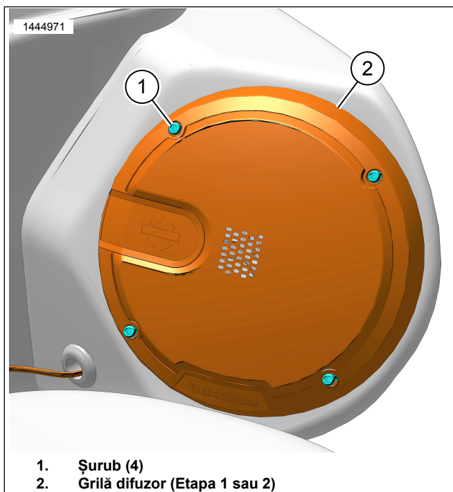
Figura 3. Grilă montură difuzor (prezentată partea stângă)
