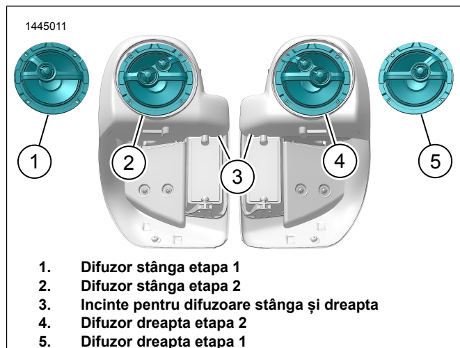
Figura 2. Orientare difuzor model Air Cooled (răcit cu aer)
