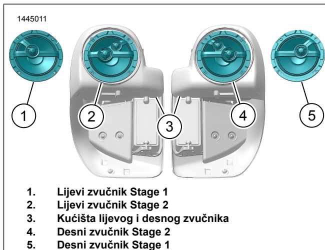
Slika 2. Orijentacija zvučnika na modelima sa zračnim hlađenjem
