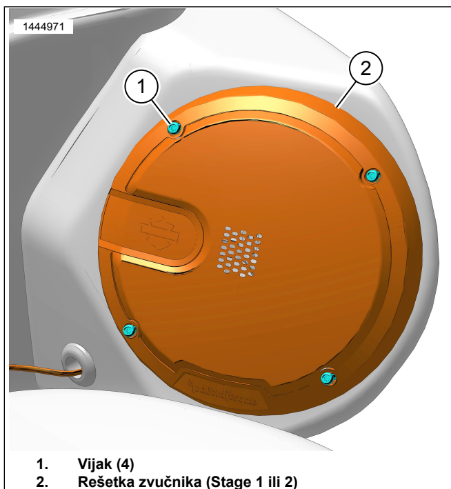
Slika 3. Rešetka zvučnika u kućištu (prikazana lijeva strana)
