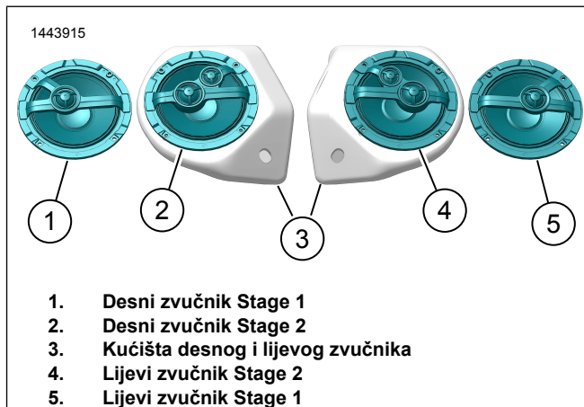
Slika 1. Orijentacija zvučnika za Tour-Pak
