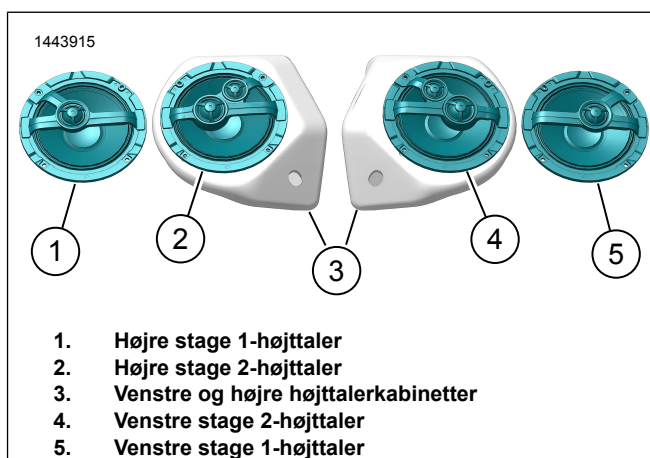
Figur 1. Tour-Pak højttalerretning
