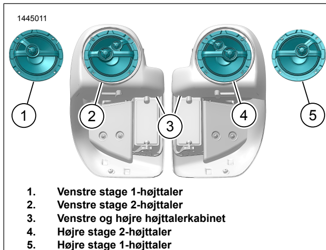
Figur 2. Luftkølet højttalerretning
