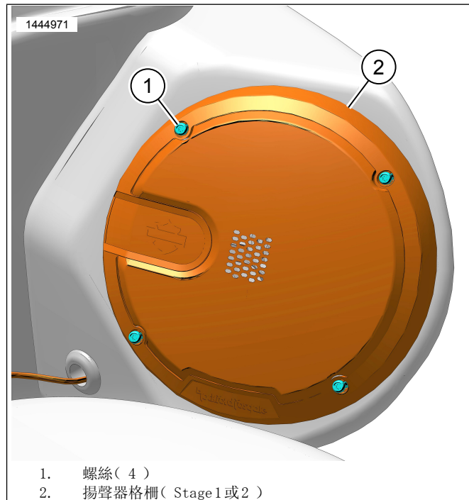
圖3。揚聲器座格柵(顯示左側)
