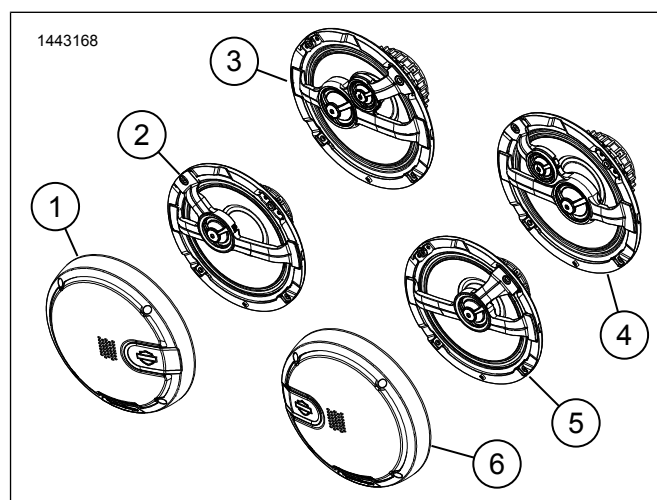
圖4。維修零件、Boom! Audio 6.5英寸後揚聲器工具包
