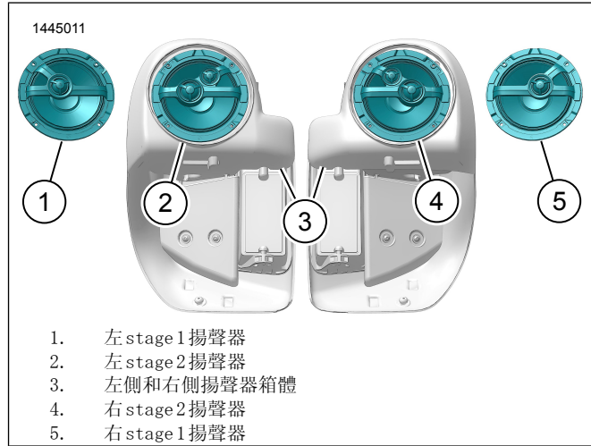
圖2。氣冷式揚聲器方向
