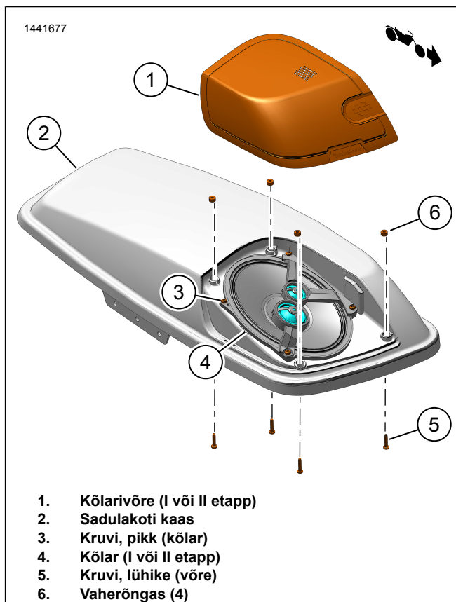
Joonis 1. Kõlari ja võre paigaldus
