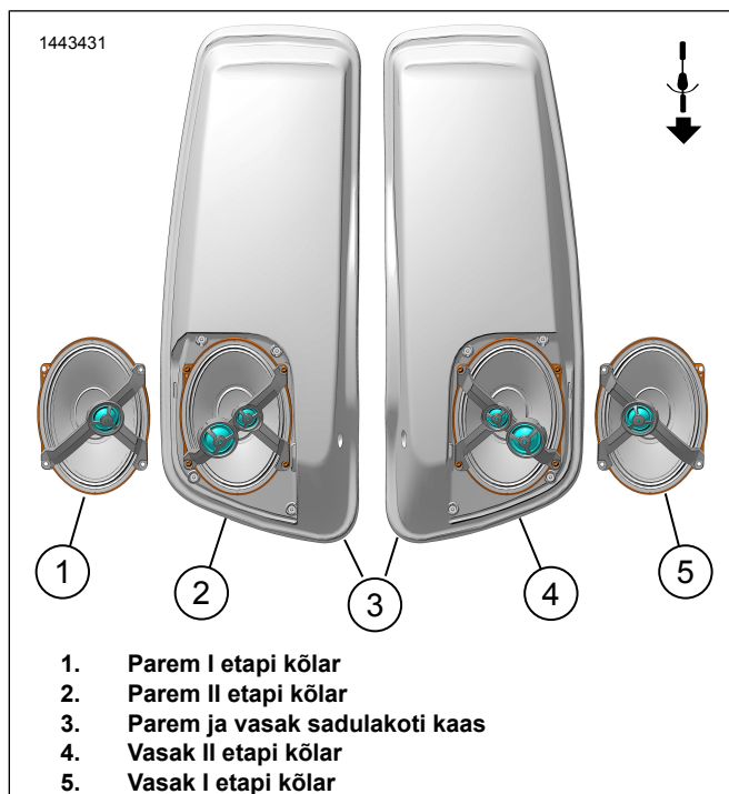
Joonis 2. Kõlari suund (tüüpiline)
