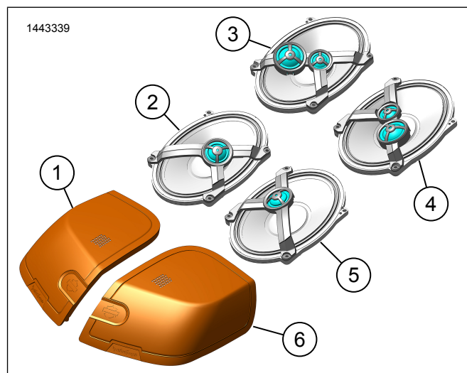
Joonis 3. Varuosad, Boom! Audio II etapi sadulakoti kõlari komplekt
