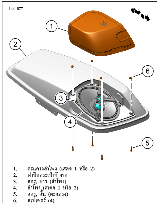
รูปภาพ 1 ติดตั้งลำโพงและตะแกรง
