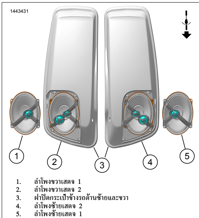
รูปภาพ 2 ทิศทางของลำโพง (ทั่วไป)
