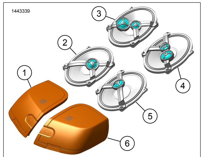
รูปภาพ 3 ชิ้นส่วนอะไหล่ ชุดลำโพงติดกระเปาะข้างรถ Boom! Audio Stage II
