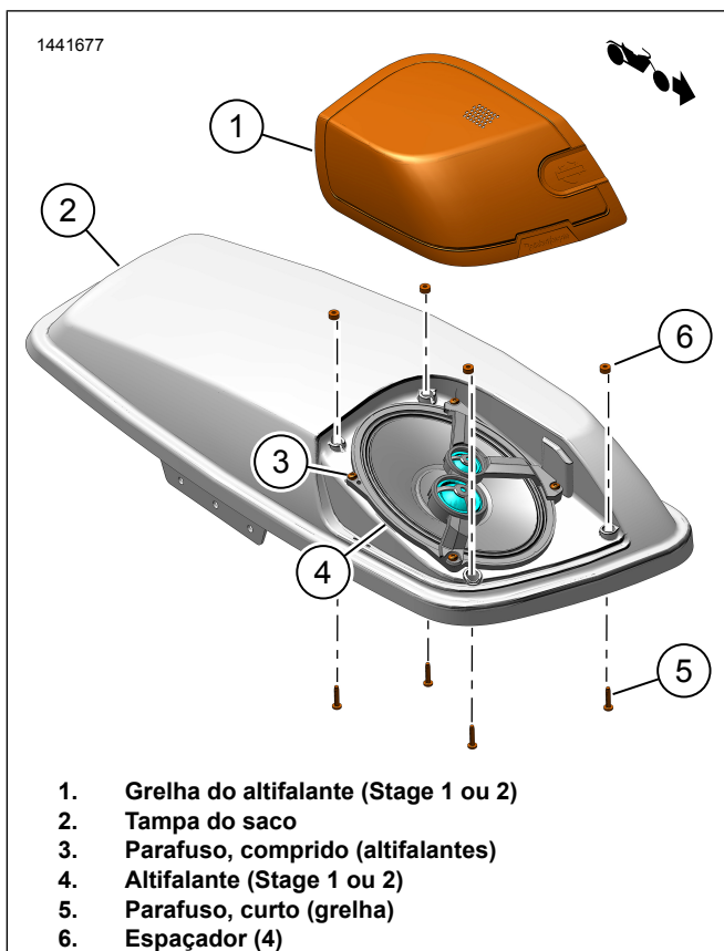
Figura 1. Instalação de altifalantes e grelha
