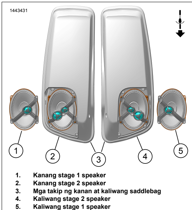
Figure 2. Oryentasyon ng Speaker (Karaniwan)
