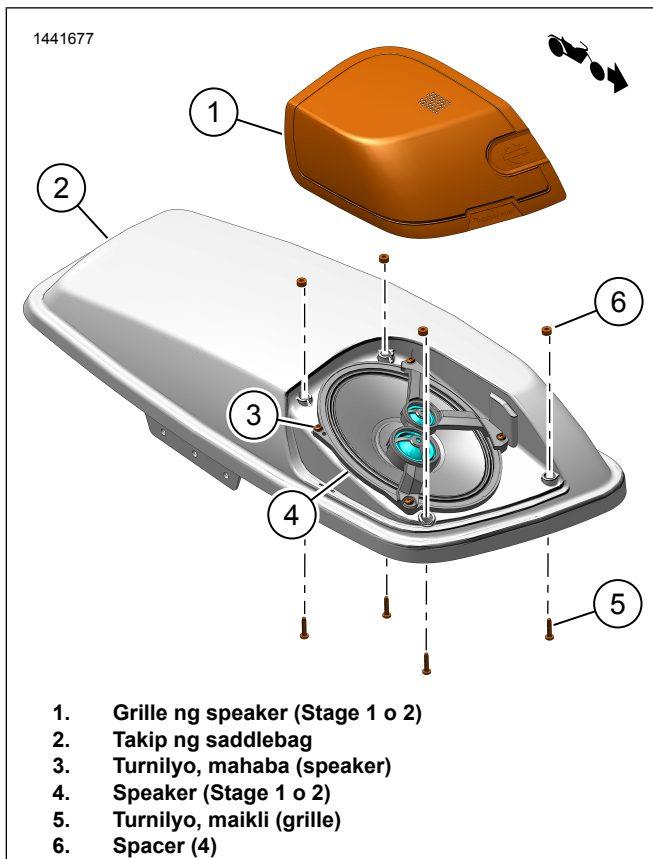
Figure 1. Pagkakabit ng Speaker at Grille
