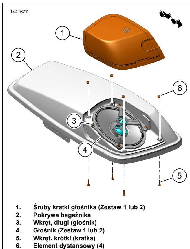
Rysunek 1. Montaż głośnika i kratki
