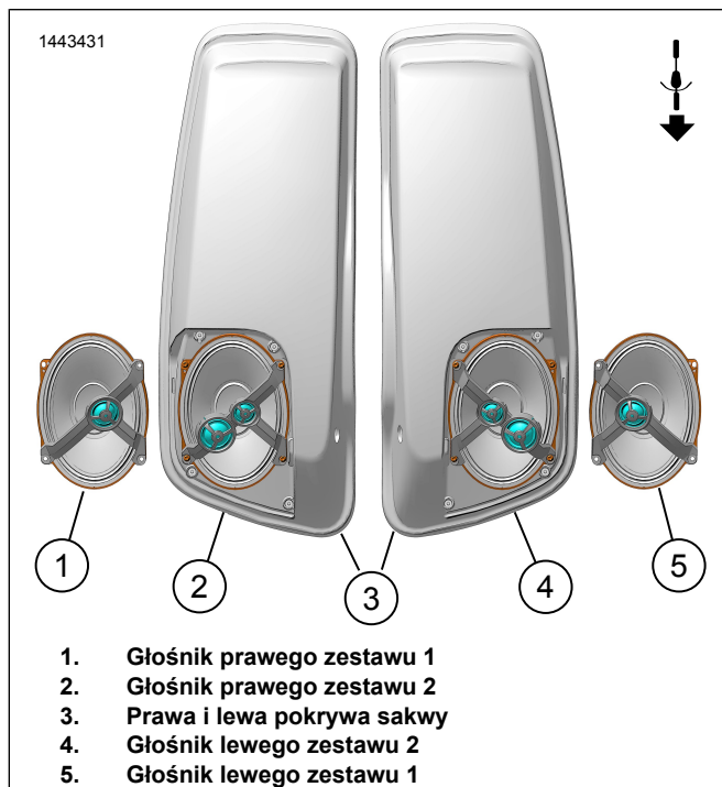
Rysunek 2. Pozycja głośnika (typowa)
