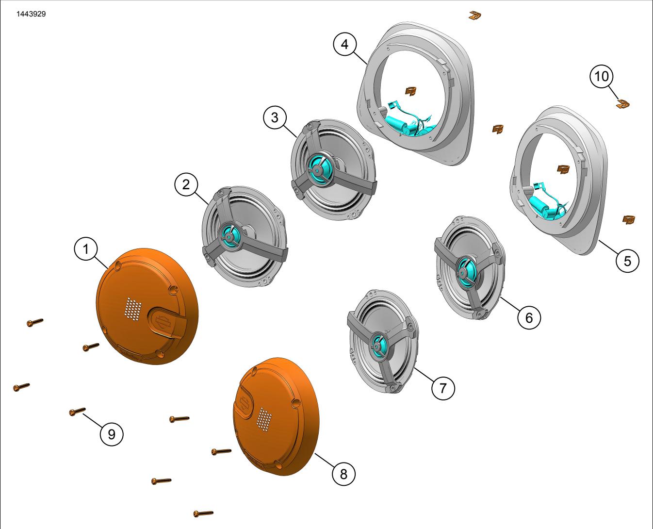
Afbeelding 4. Serviceonderdelen, Onderkuipluidsprekers
