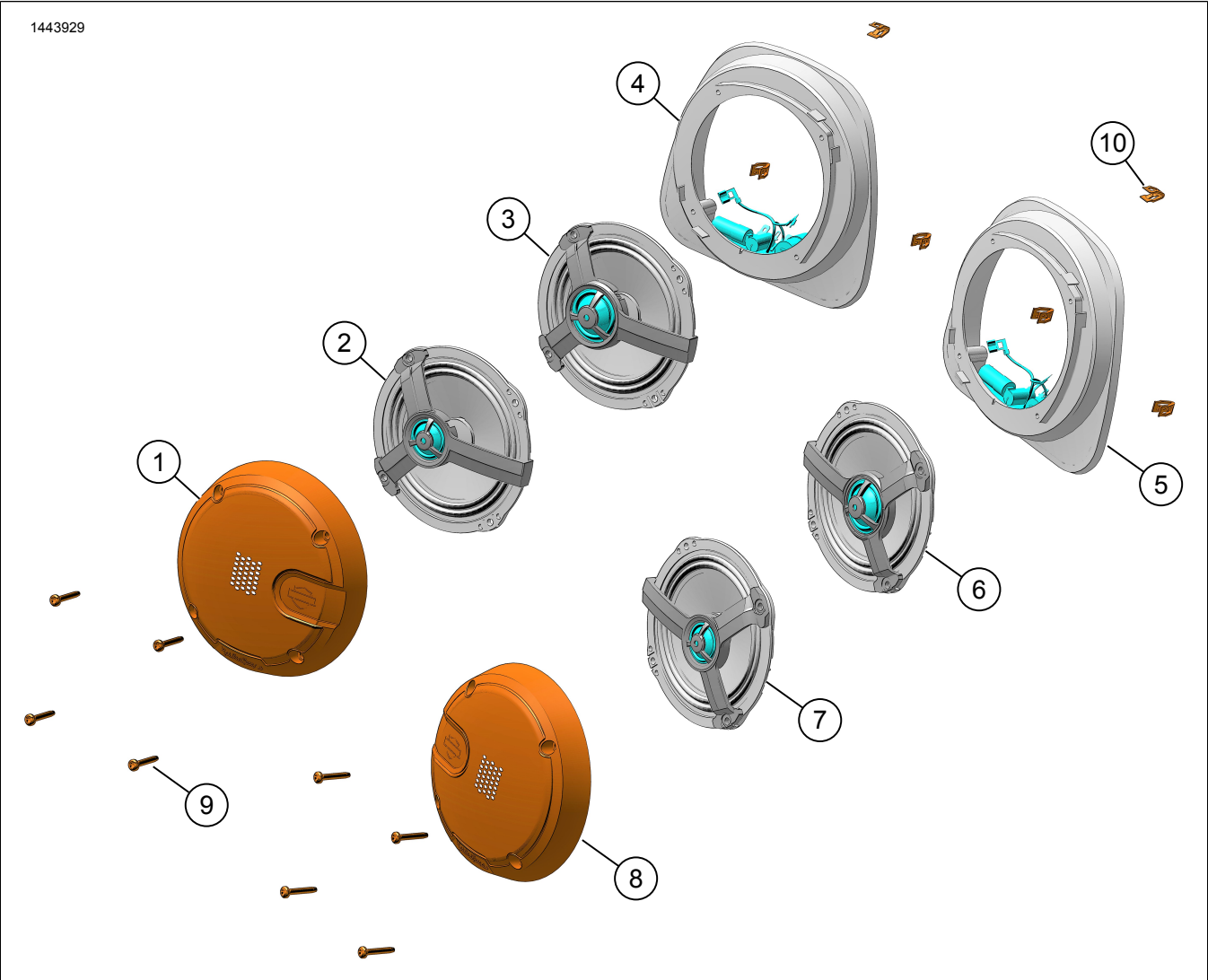
Slika 4. Servisni dijelovi, zvučnici u donjoj maski
