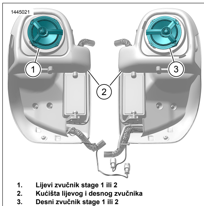
Slika 3. Orijentacija zvučnika na modelima s dvostrukim hlađenjem
