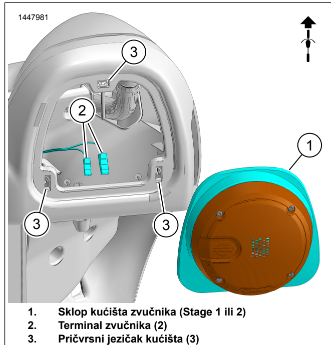
Slika 2. Ugradnja zvučnika za donju masku
