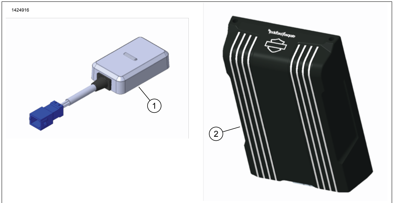
Figure 1. Pièces de rechange : Kit amplificateur primaire
