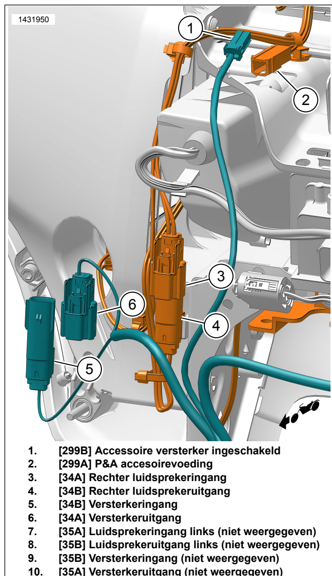
Afbeelding 1. Op vork gemonteerde luidsprekerkabelboom (rechterkant getoond, links vergelijkbaar)
