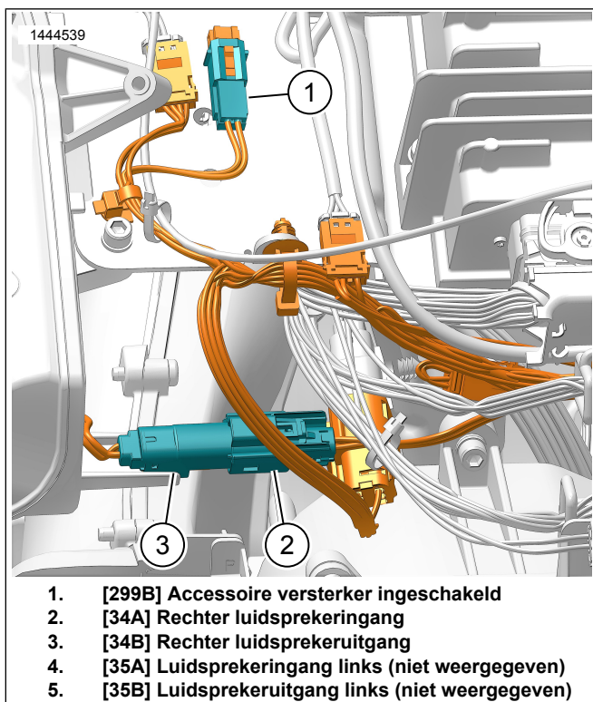
Afbeelding 2. Op frame gemonteerde luidsprekerkabelboom (rechterkant getoond, links vergelijkbaar)
