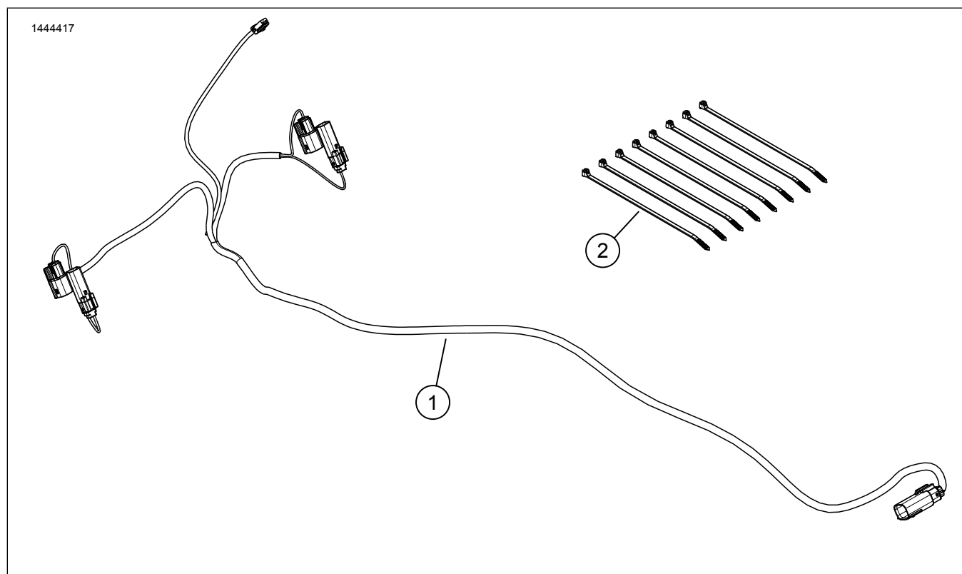
Afbeelding 4. Serviceonderdelen, versterkermontageset
