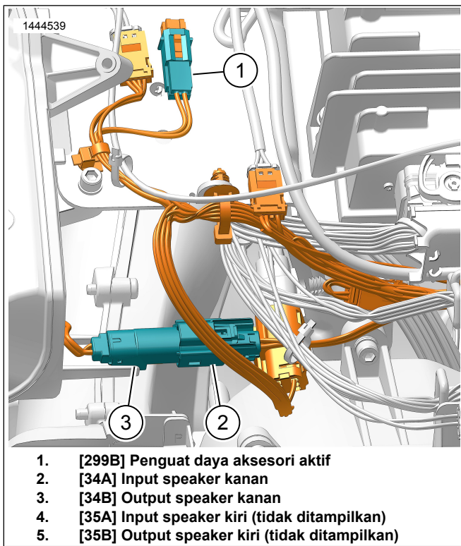
Gambar 2. Harness Speaker Terpasang Pada Rangka (Sisi Kanan Ditampilkan, Bagian Kiri Sama)
