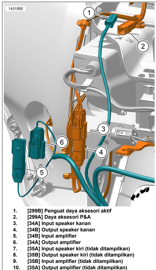
Gambar 1. Harness Speaker Terpasang Pada Garpu (Sisi Kanan Ditampilkan, Bagian Kiri Sama)
