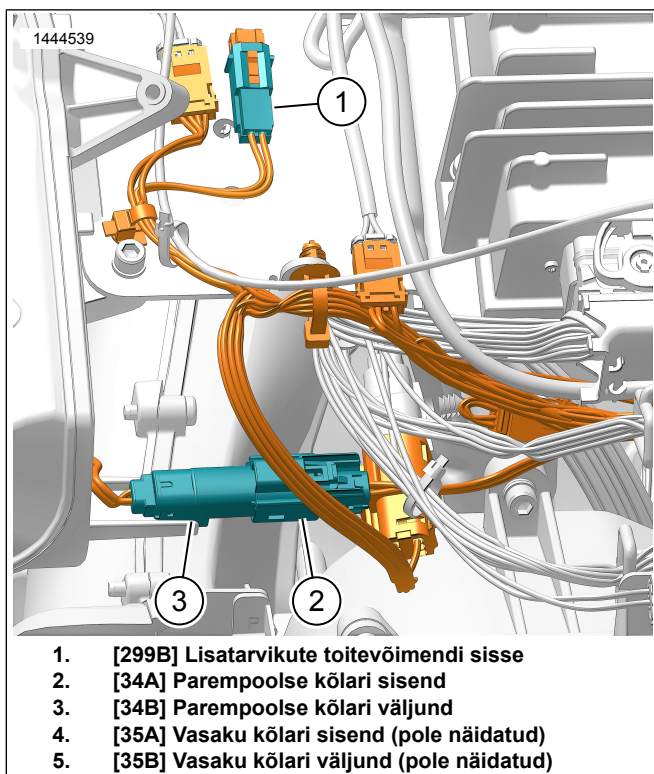
Joonis 2. Raamile paigaldatav kõlarijuhtmestik (näidatud parempoolne, vasakpoolne on sarnane)
