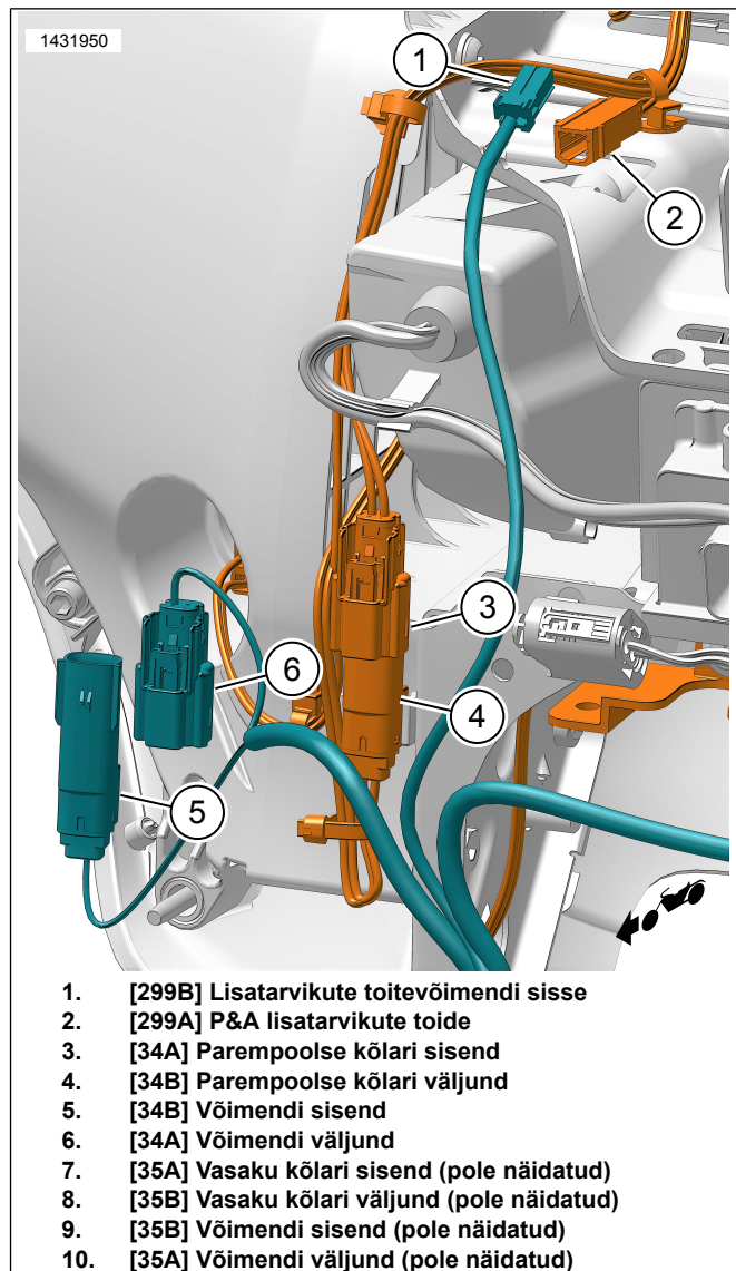
Joonis 1. Kahvli paigaldatav kõlarijuhtmestik (näidatud parempoolne, vasakpoolne on sarnane)
