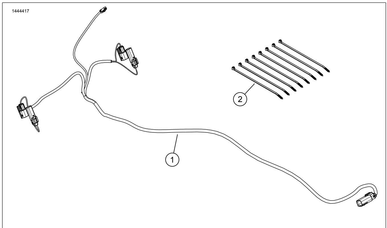
Joonis 4. Varuosad, võimendi paigalduskomplekt
