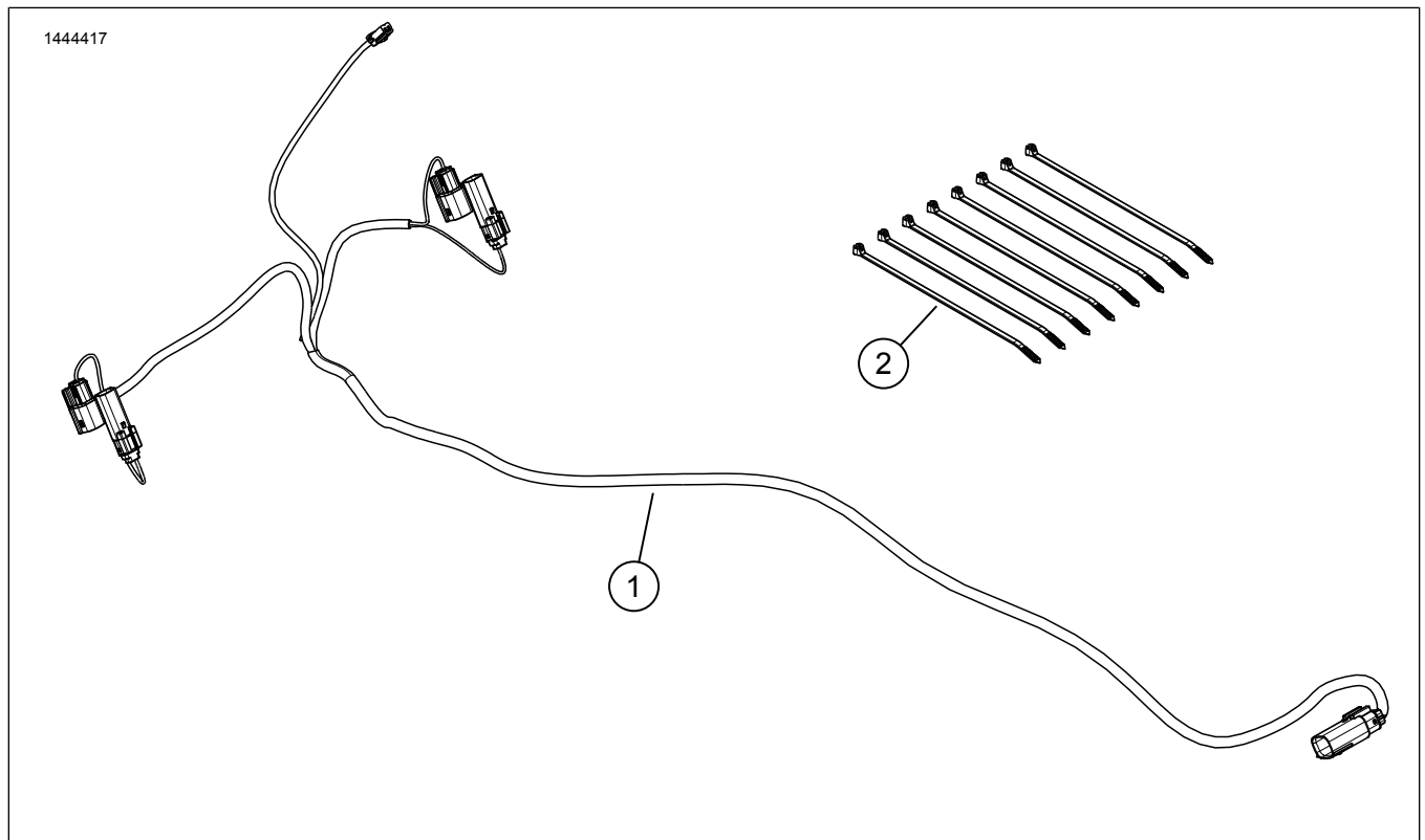
Figur 4. Servicedelar, installationssats för förstärkare
