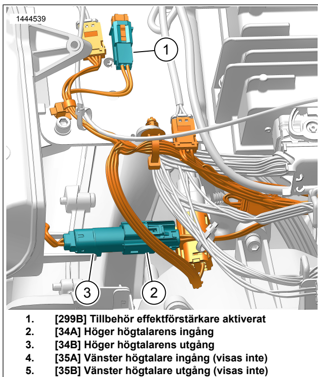
Figur 2. Rammonterat högtalares kablage (höger sida visad, vänster liknande)
