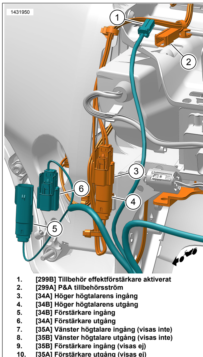
Figur 1. Gaffelmonterat högtalares kablage (höger sida visad, vänster liknande)
