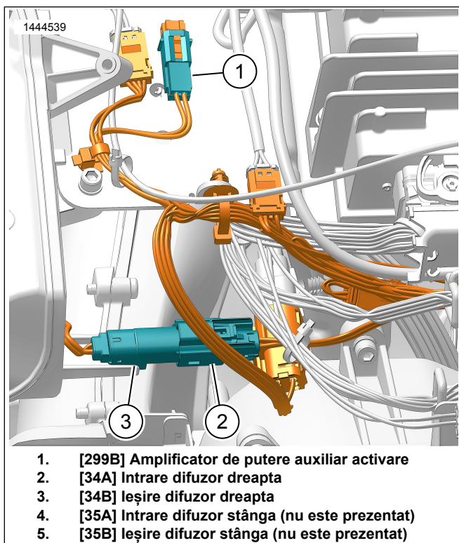
Figura 2. Cablaj difuzor montat pe cadru (partea dreaptă prezentată, partea stângă similară)
