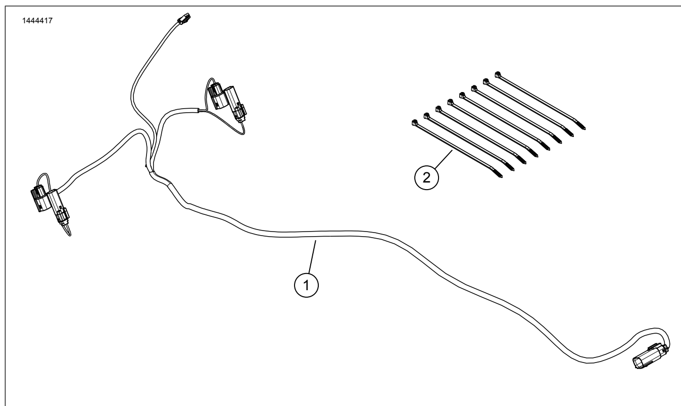
Figura 4. Kit de instalare amplificator, componente de service
