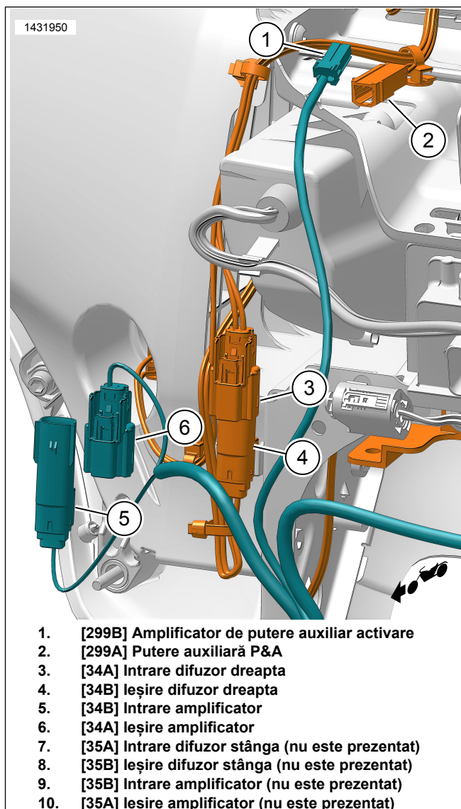
Figura 1. Cablaj difuzor montat pe furcă (partea dreaptă prezentată, partea stângă similară)
