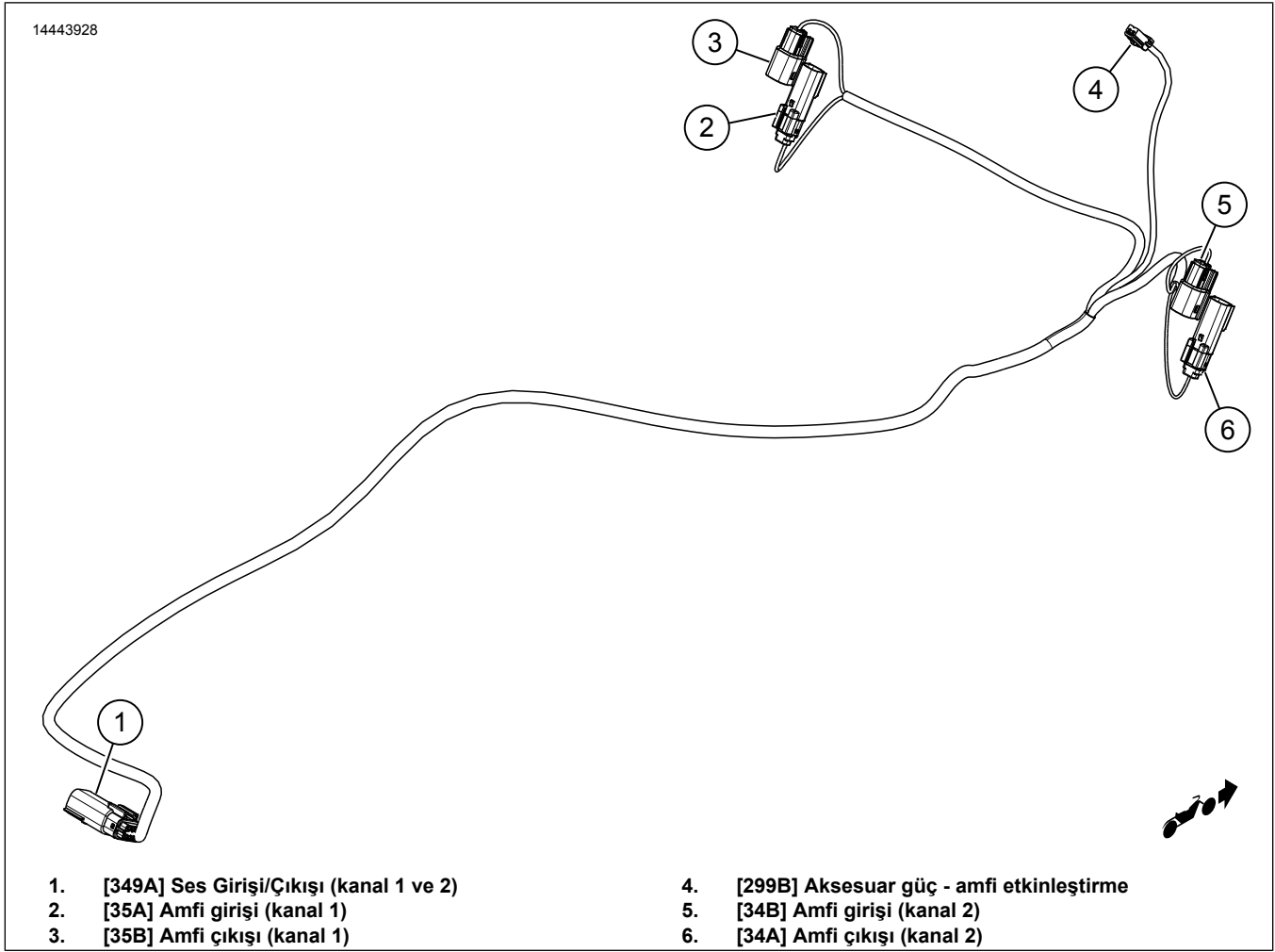
Şekil 3. Kaporta Hoparlörü Kablo Takımı
