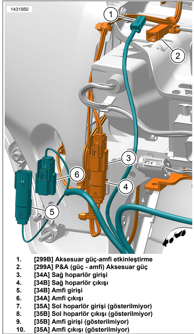
Şekil 1. Çatala Monte Hoparlör Kablo Takımı (Sağ Taraf Gösteriliyor, Sol da Aynıdır)
