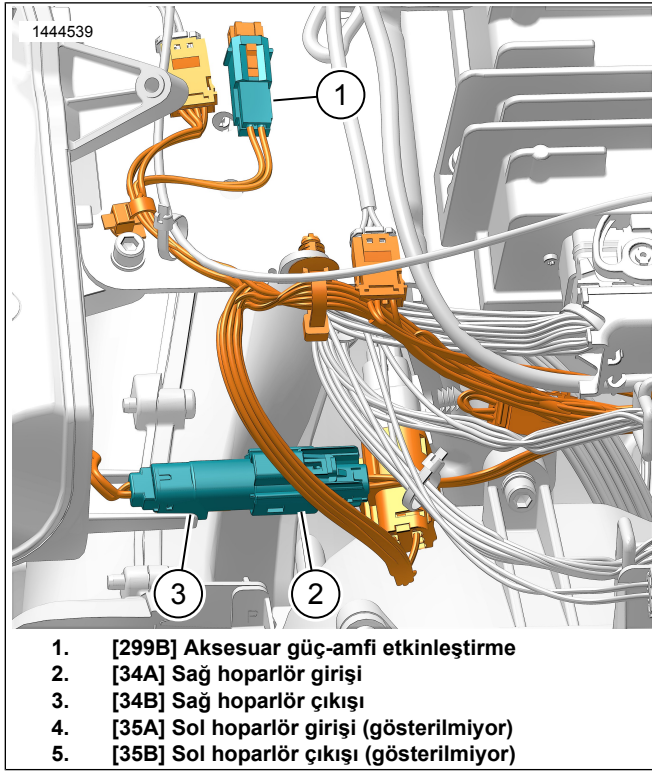
Şekil 2. Şasiye Monte Hoparlör Kablo Takımı (Sağ Taraf Gösteriliyor, Sol da Aynısı)
