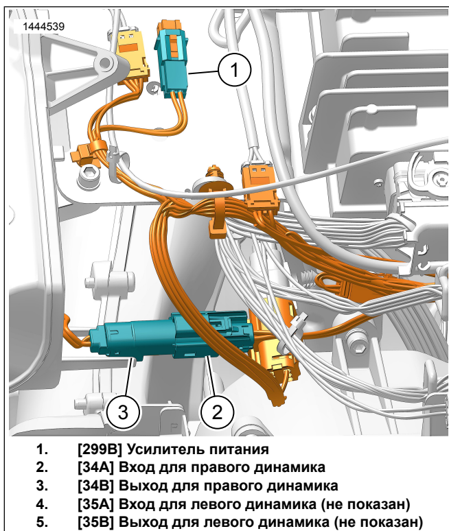
Рисунок 2. Жгут устанавливаемого на раму динамика (показана правая сторона, левая сторона такая же)
