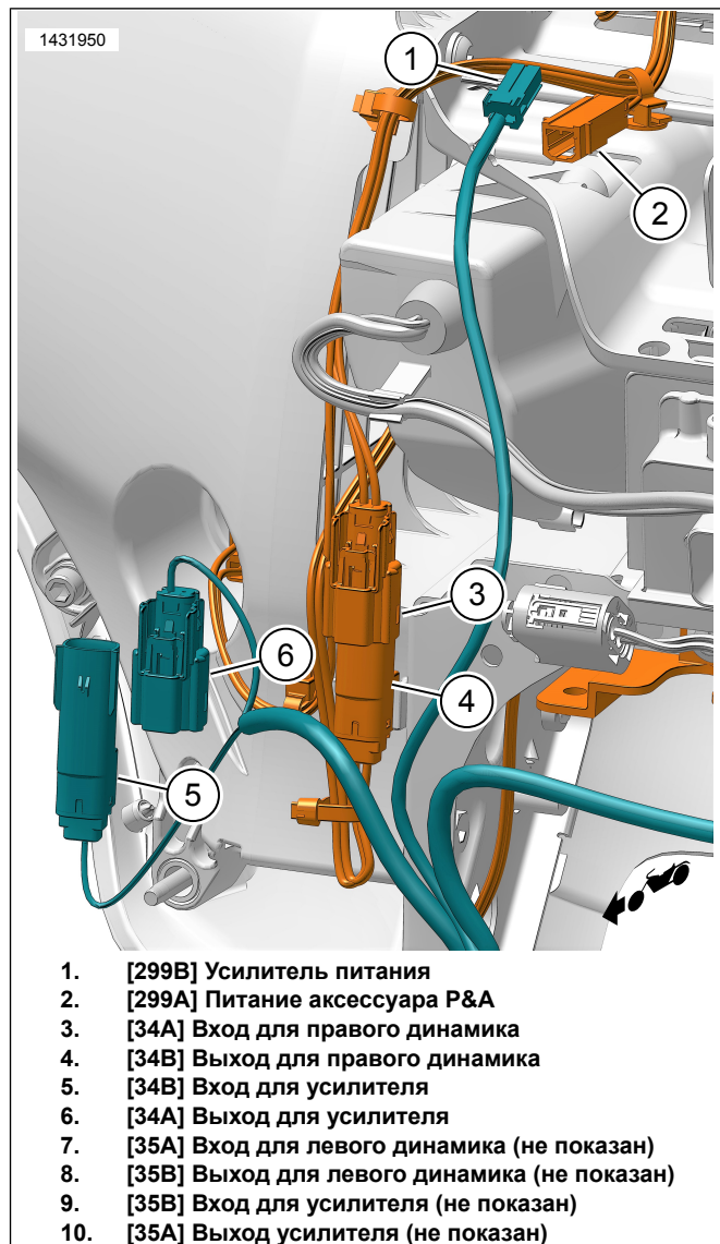
Рисунок 1. Жгут закрепляемого на вилке динамика (показана правая сторона, левая сторона такая же)
