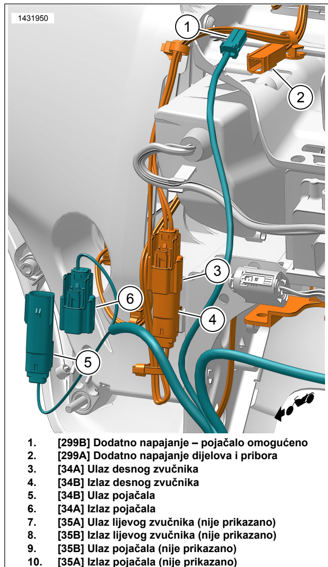
Slika 1. Kabelski snop zvučnika montiranih na vilicu (prikazana desna strana, na lijevoj je slično)
