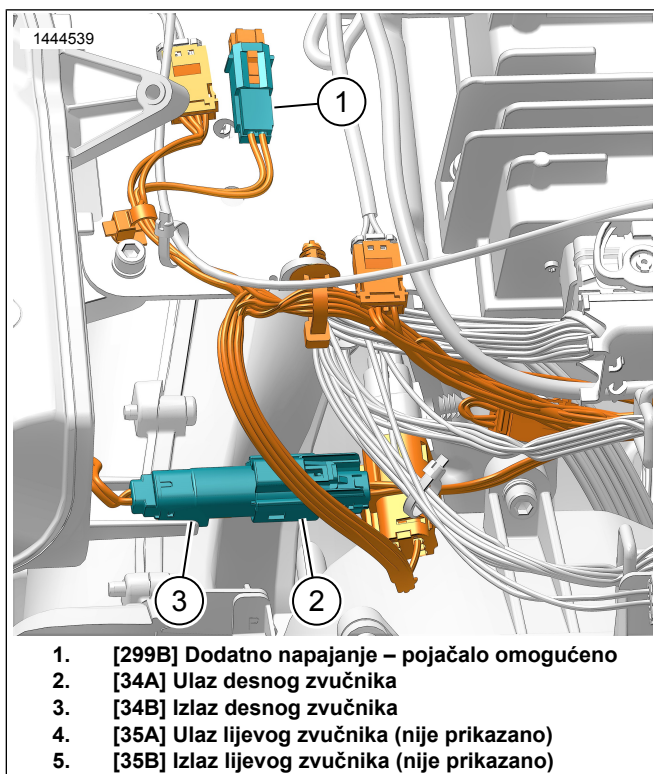
Slika 2. Kabelski snop zvučnika montiranih na okvir (prikazana desna strana, na lijevoj je slično)
