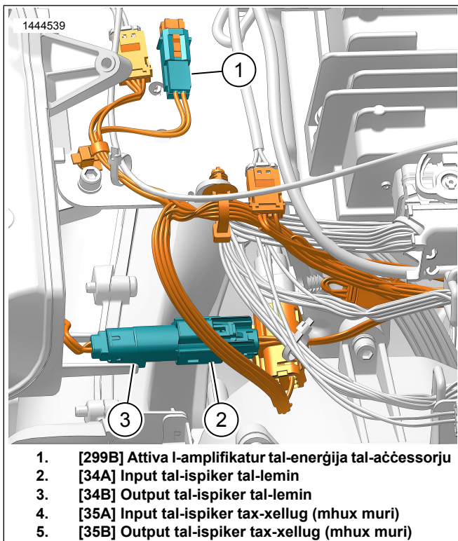
Figura 2. Harness tal-Ispiker Immuntat fuq il-Furketta (Murija n-Naħa tal-Lemm, tax-Xellug Simili)
