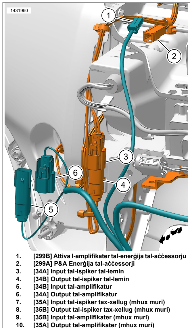
Figura 1. Harness tal-Ispeaker Immuntat fuq il-Furketa (Murija n-Naħa tal-Lemin, tax-Xellug Simili)
