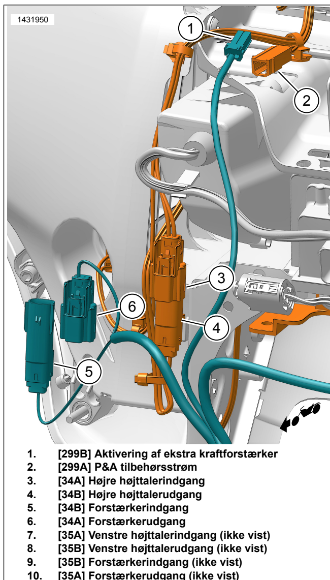
Figur 1. Gaffelmonteret højttalerledning (højre side vist, venstre er magen til)
