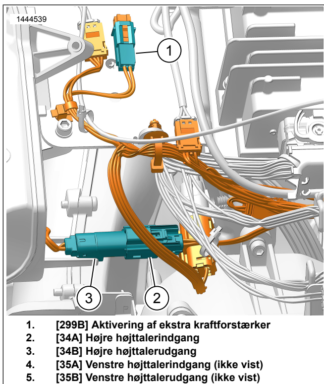
Figur 2. Stelmonteret højtalerledning (højre side vist, venstre er magen til)
