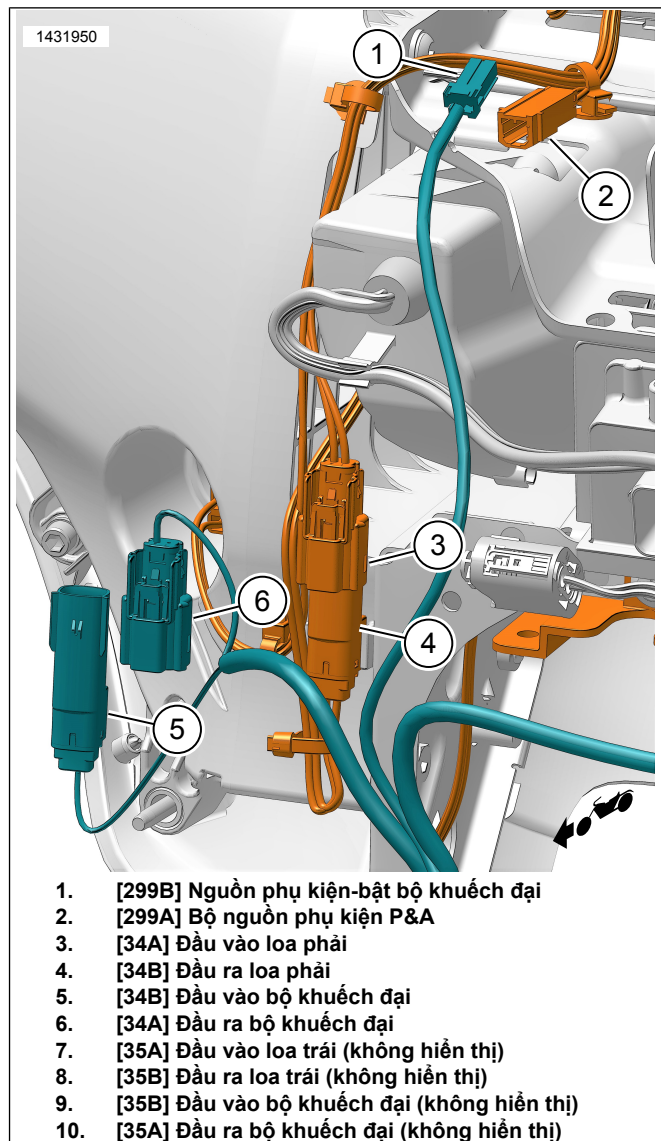
Hình 1. Bó dây Loa lắp ở phụộc (Minh hoạ bên phải, bên trái tương tự)
