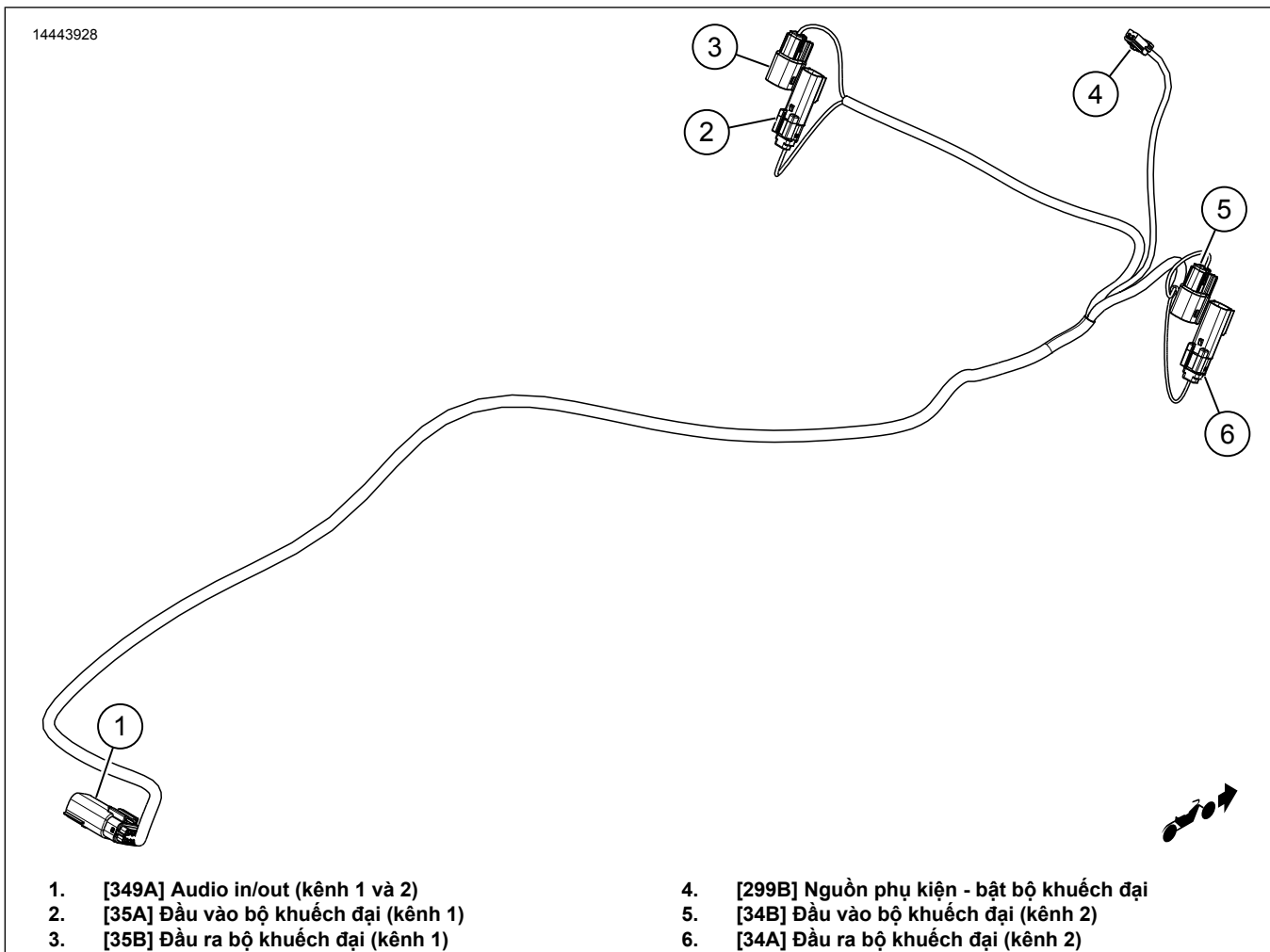
Hình 3. Bó dây loa yếm xe
