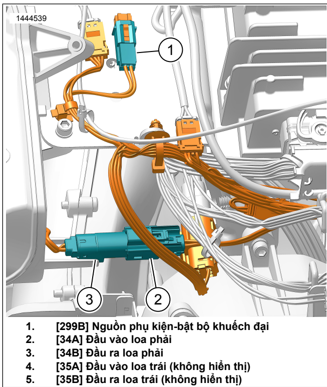
Hình 2. Bó dây Loa lắp ở khung (Minh hoạ bên phải, bên trái tương tự)
