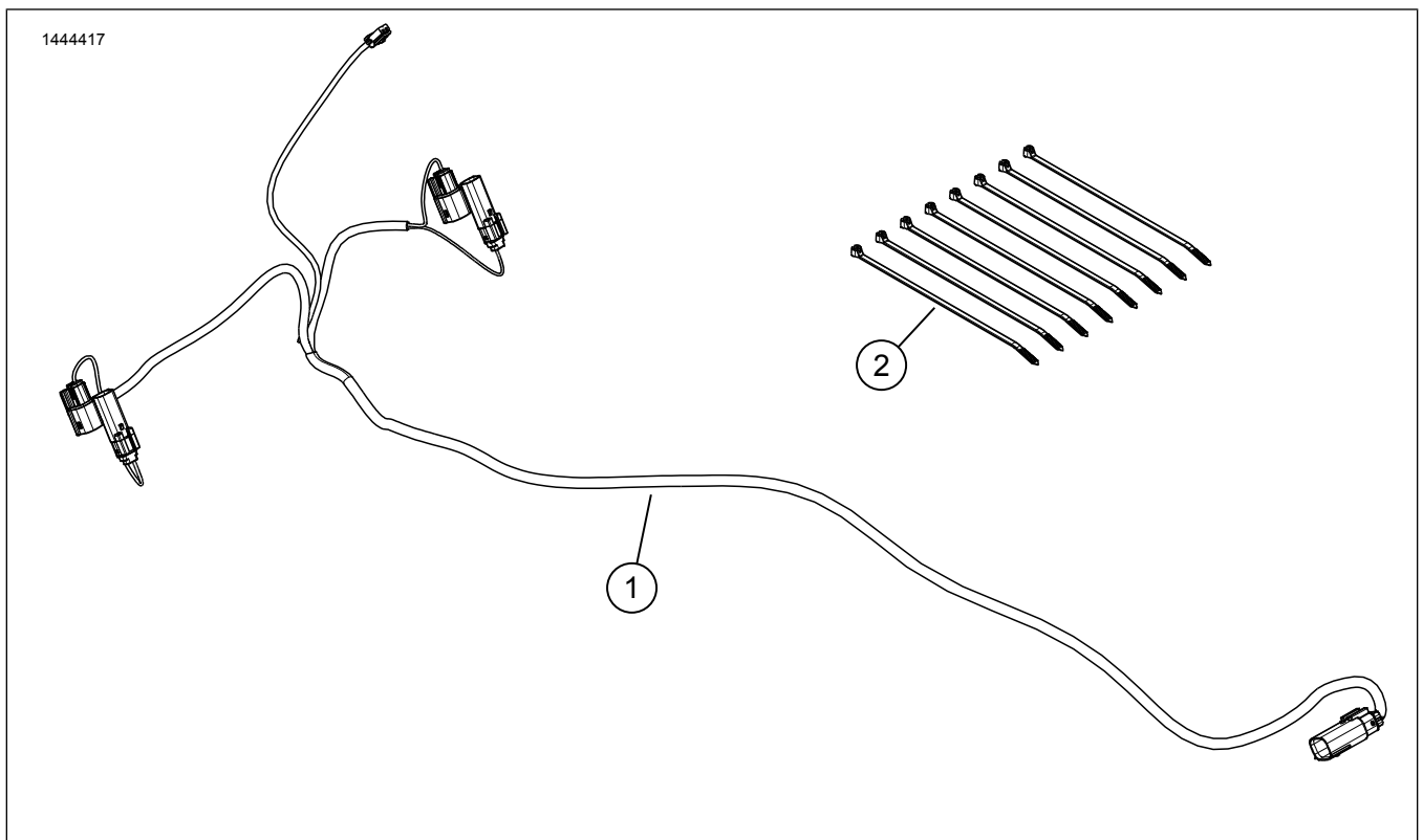
Hình 4. Phụ tùng dịch vụ, Bộ lắp đặt bộ khuếch đại
