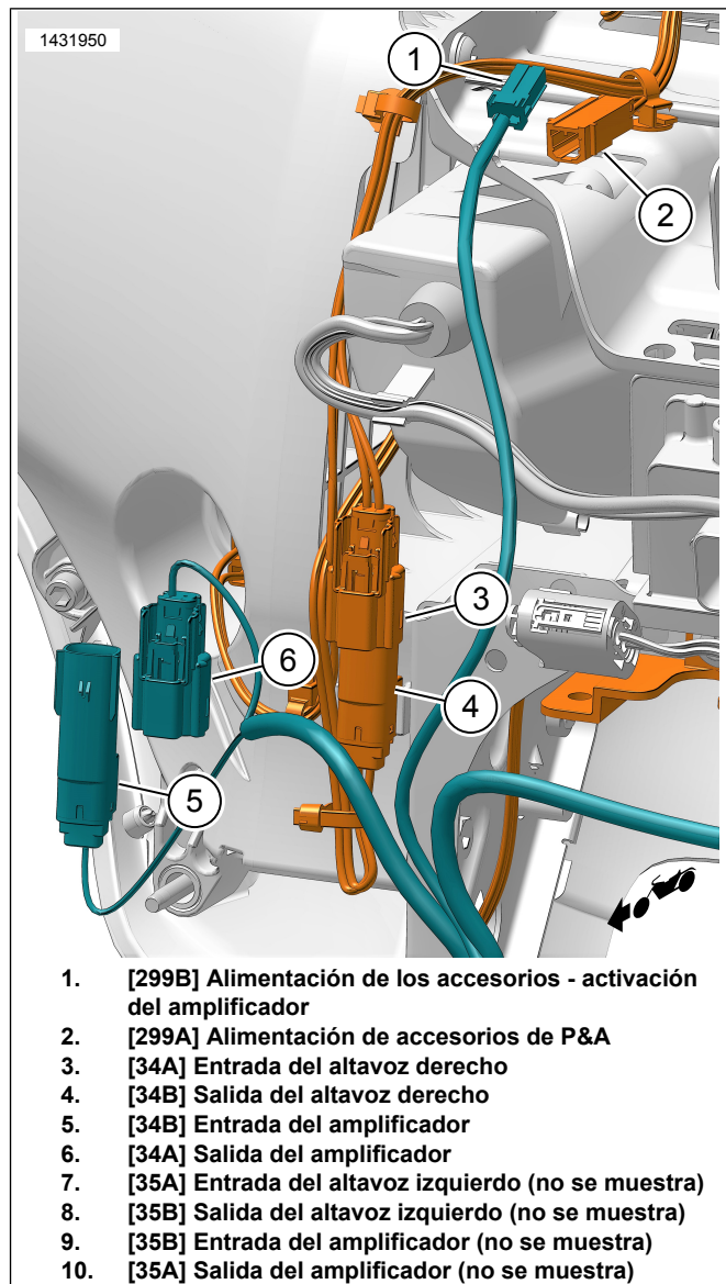
Figura 1. Arnés de altavoz montado en la horquilla (se muestra en el lado derecho, similar en el lado izquierdo)
