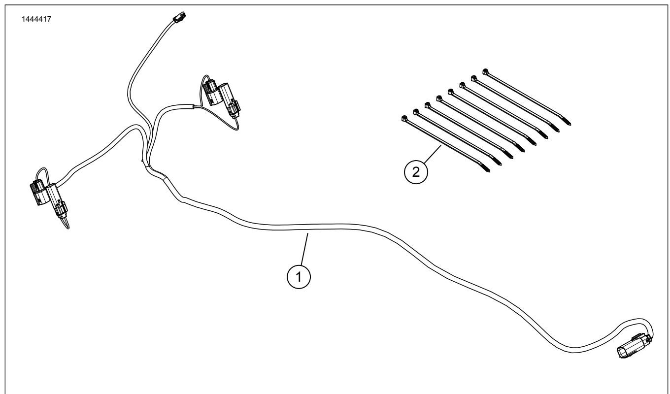
Figura 4. Piezas de servicio, kit de instalación del amplificador
