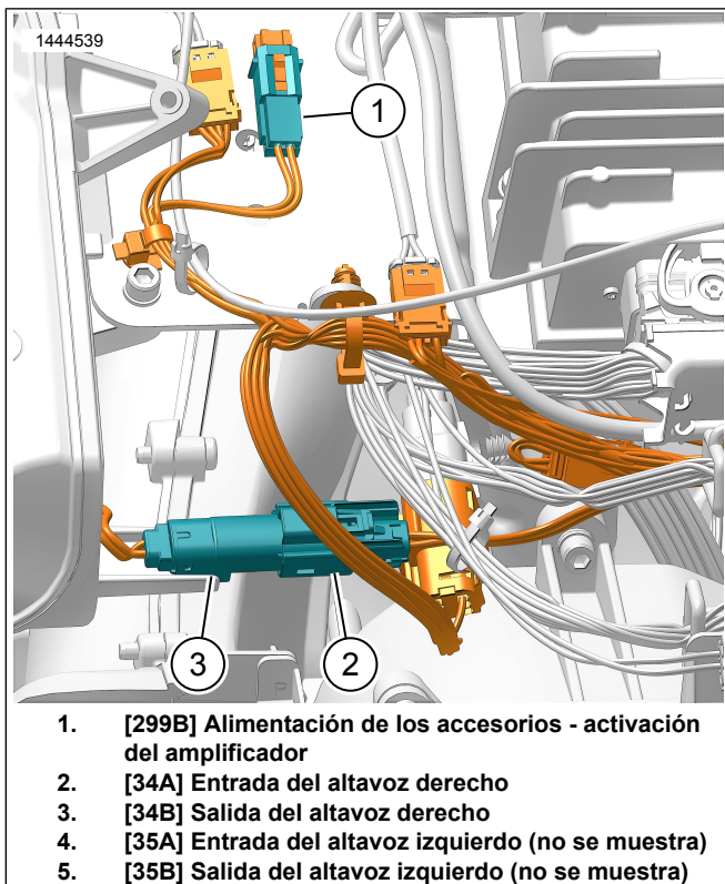
Figura 2. Arnés de altavoz montado en la estructura (se muestra en el lado derecho, similar en el lado izquierdo)
